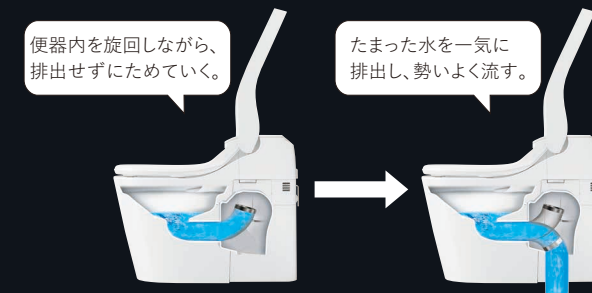
ターントラップ方式 パナソニック独自の排水機構。 少ない水で一気に流しきる。
