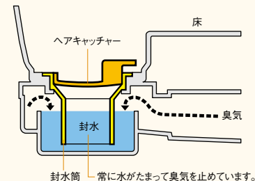
●排水トラップ断面図
