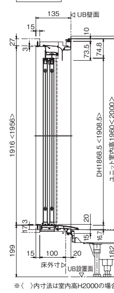
ドア部断面図
