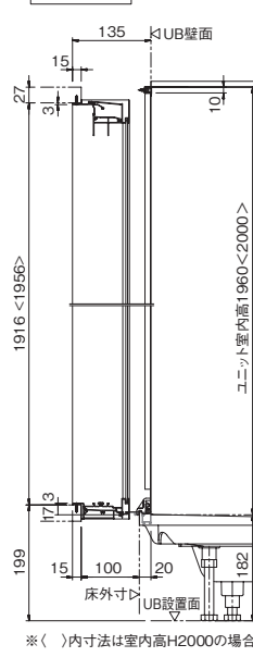
戸袋部断面図
