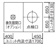
天井伏図
