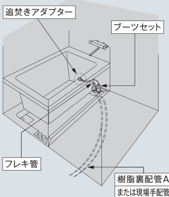
通常納まり仕様(正面)
