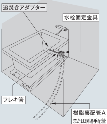
壁納まり仕様
