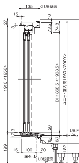
ドア部断面図
