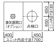
天井伏図
