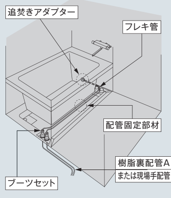
スリム納まり仕様(手前)
