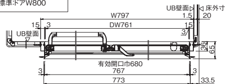
ドア幅100カット(ドアコーナー寄せ)
