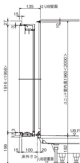
戸袋部断面図
