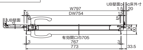
標準ドアW800
