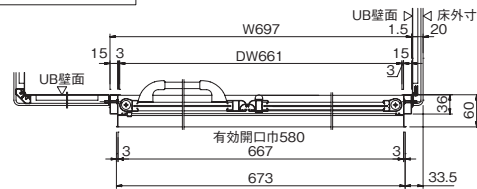
ドア幅100カット(ドアコーナー寄せ)
