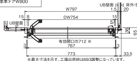
ドア幅100カット(ドアコーナー寄せ)
