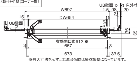
ドア幅100カット+小壁(コーナー側)
