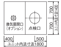
天井伏図
