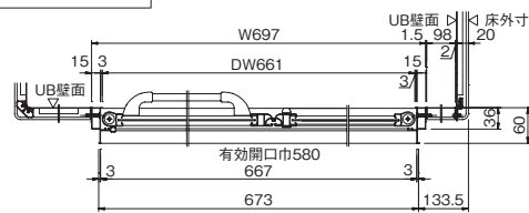
ドア幅100カット+小壁(コーナー側)
