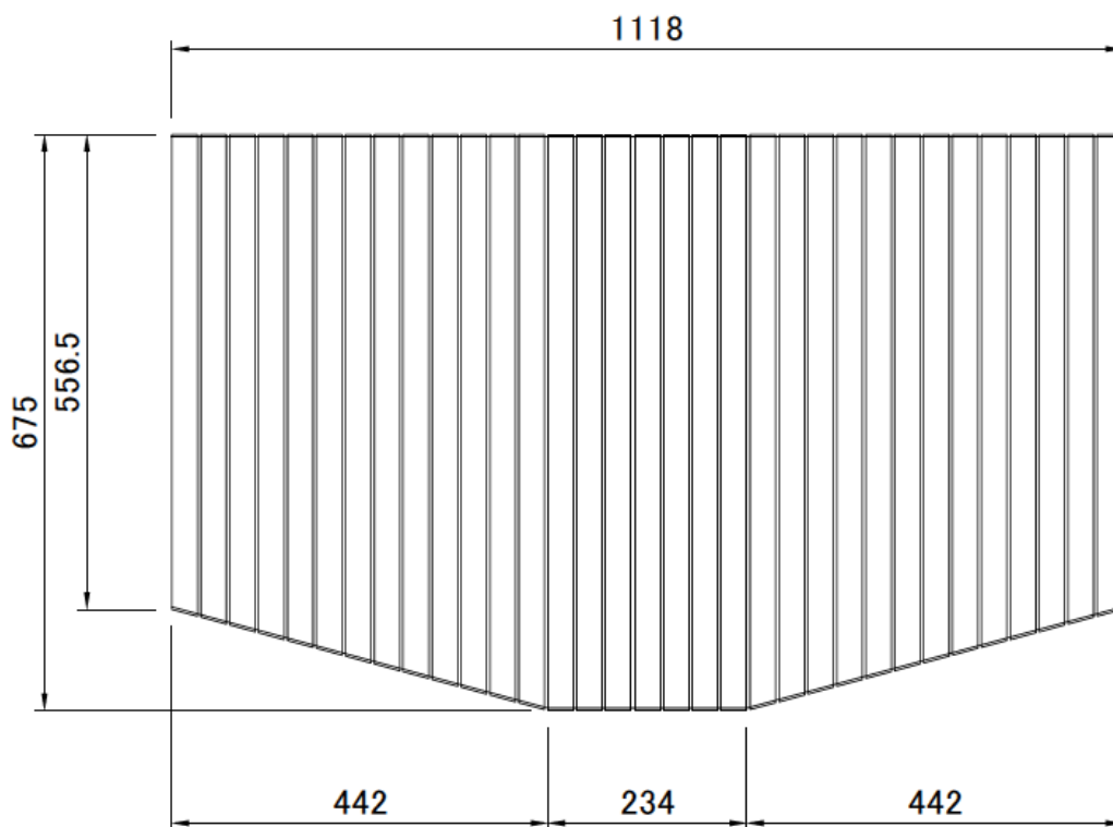
旧仕様形状
