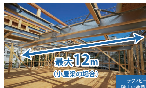
グランドテクノビーム施工例
