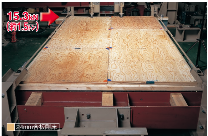
●剛床仕様(根太なし) 梁の上に根太を乗せる形となる転ばし根太と異なり、テクノビームの上に24mmの構造用合板を直接施工。床板と梁がより強固に一体化し、高強度を実現します。
