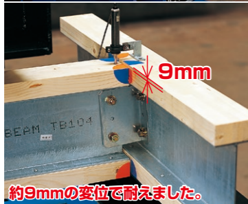
テクノビーム4.5のボルト接合
