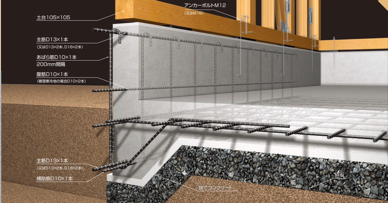
※イラストはイメージです。配筋仕様や地業工事(捨てコンクリート砕石)は、条件によって異なる場合があります。
