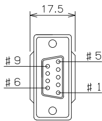
DSUB9ピン
