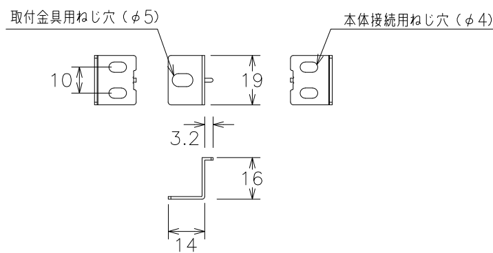
取付金具 (付属)
