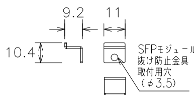
SFPモジュール抜け防止金具 (付属)
