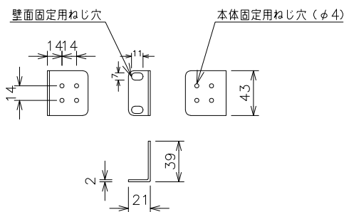
取付金具（壁取付用）（同梱）
