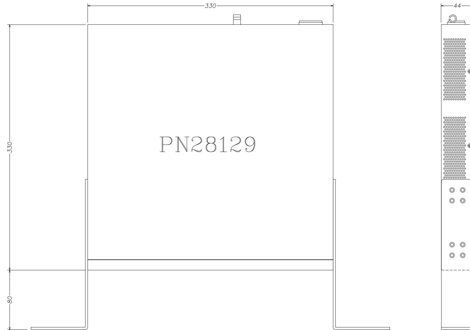
取付図 (例)
