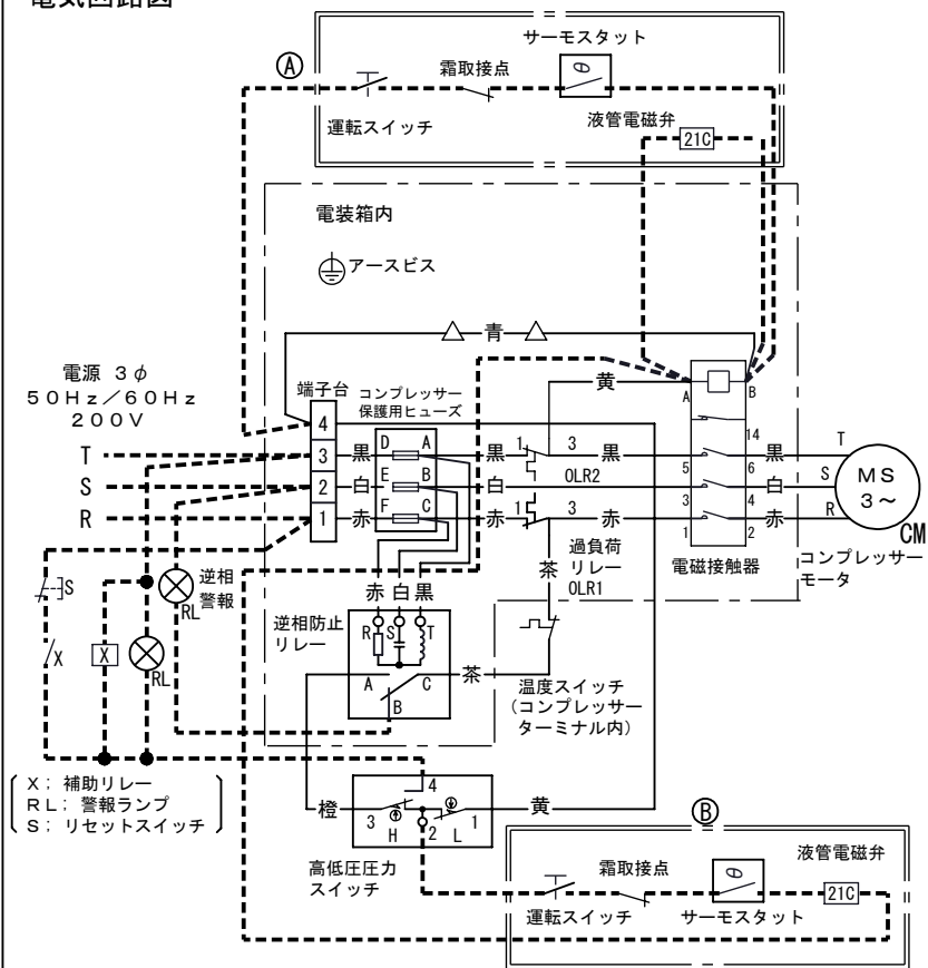
電気回路図
