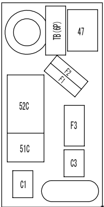
電装箱内部品配置図
