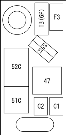
電装箱内部品配置図
