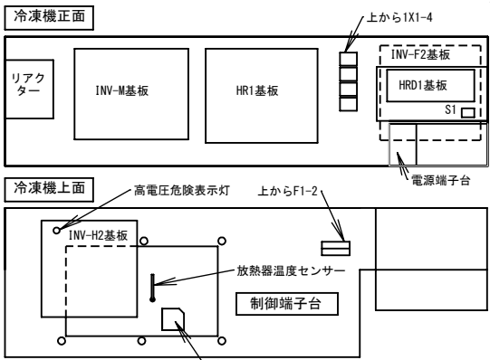
電装箱内部部品配置図
