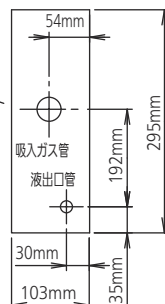
冷凍機下面配管用穴 詳細
