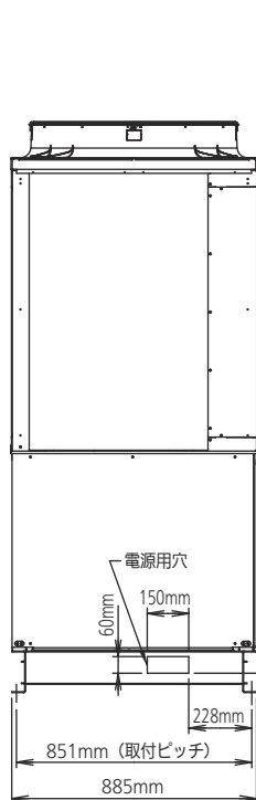
冷凍機左側面
