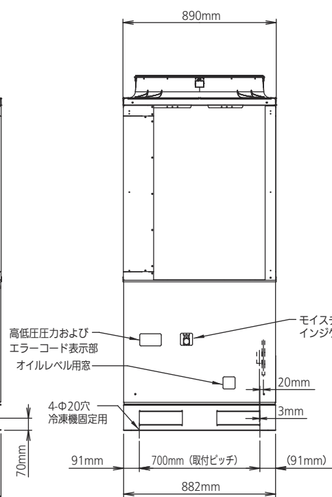
冷凍機正面
