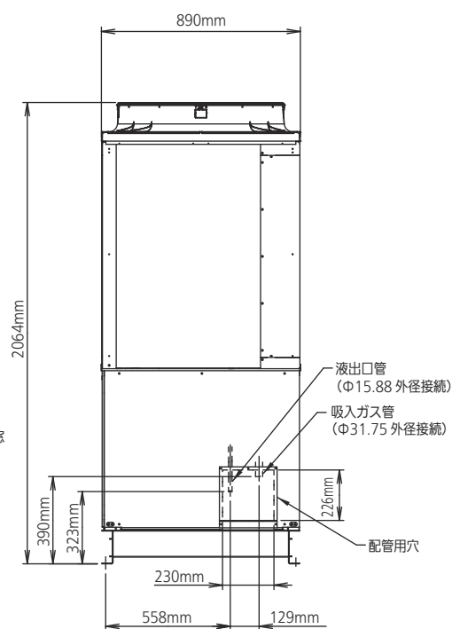
冷凍機右側面
