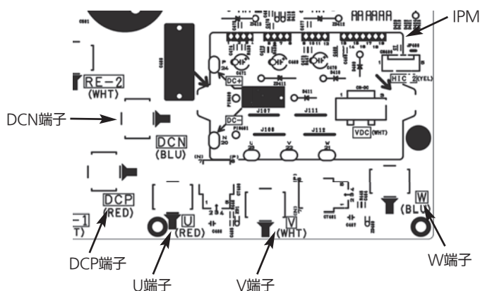
インバーター基板 (INV-H基板) 端子配列
