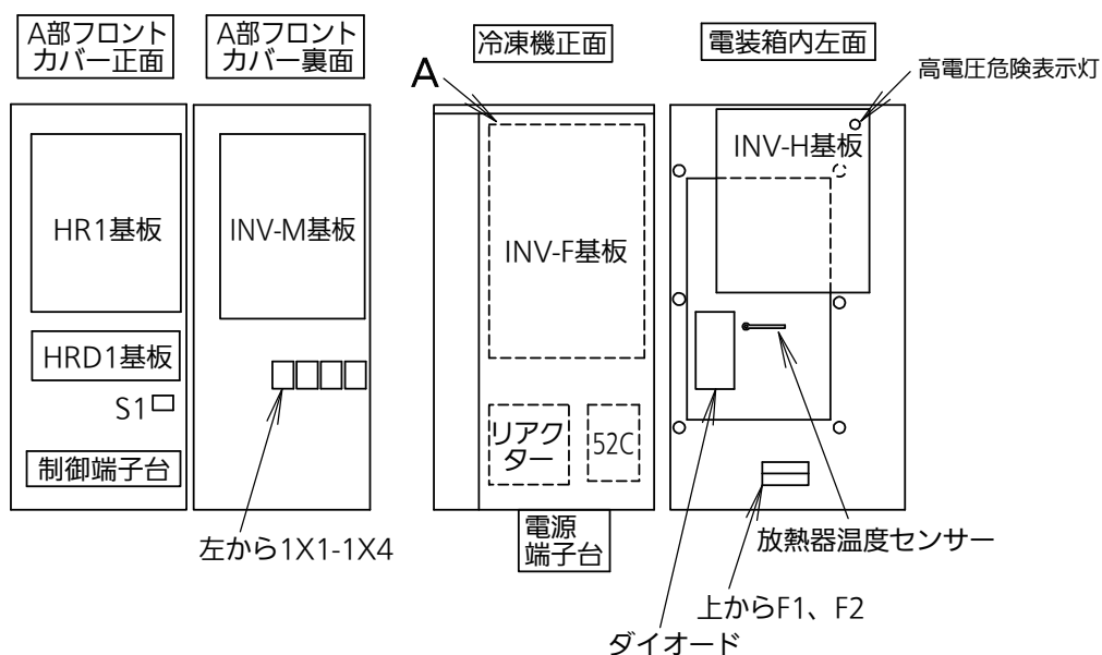
電装箱内部配置図
