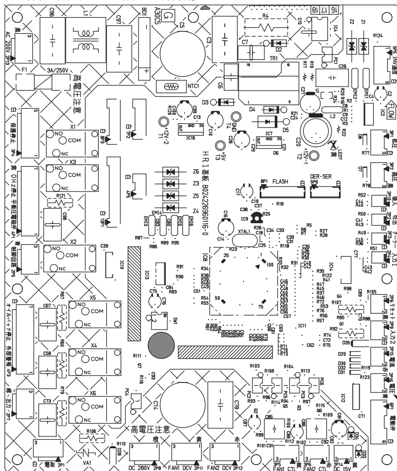
<制御基板（HRD1基板）>設定用
