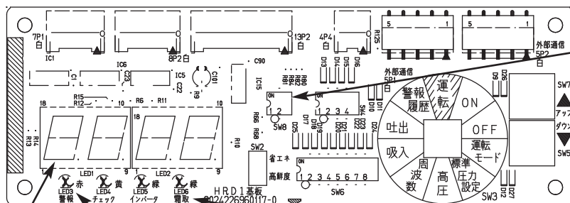
<制御基板（HRD1基板）>設定用
