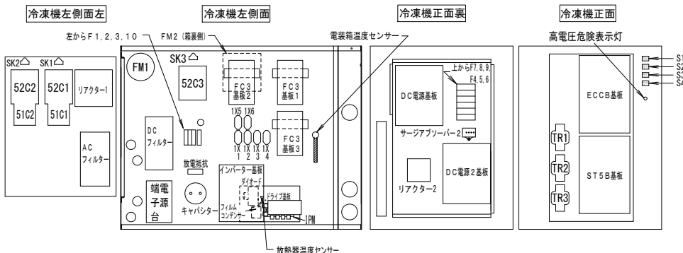
電装箱内部部品配置図
