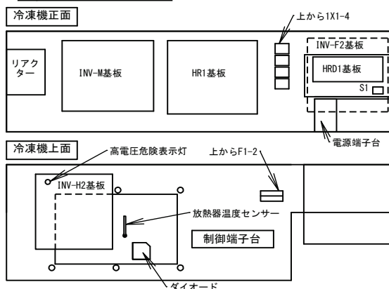
電装箱内部部品配置図
