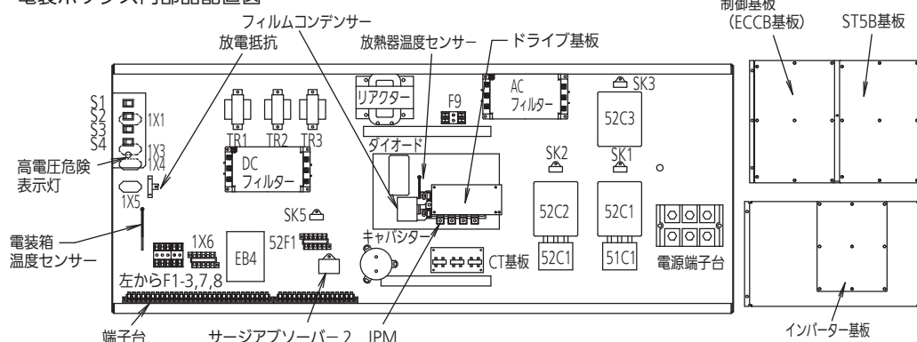
電装ボックス内部品配置図
