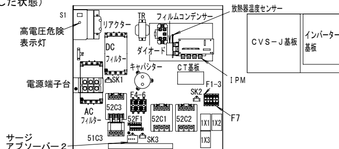
電装箱内部部品配置図 (基板を外した状態)
