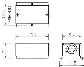
ターミナルボックス (付属品)
