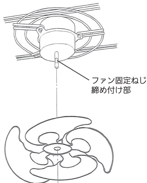
吐出タイプのファン取り付け状態
