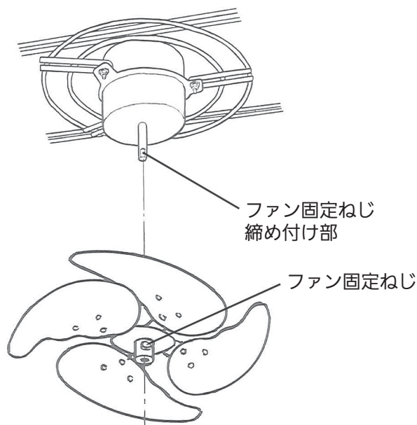
吸込タイプ（出荷時）のファン取り付け状態
