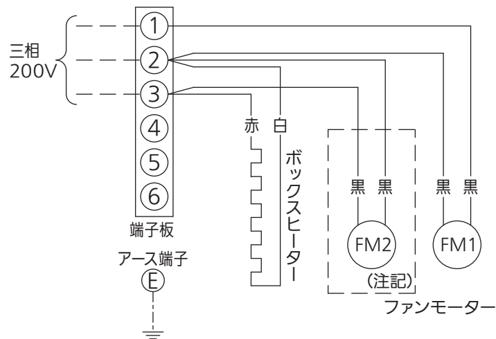
冷蔵用電気回路図
