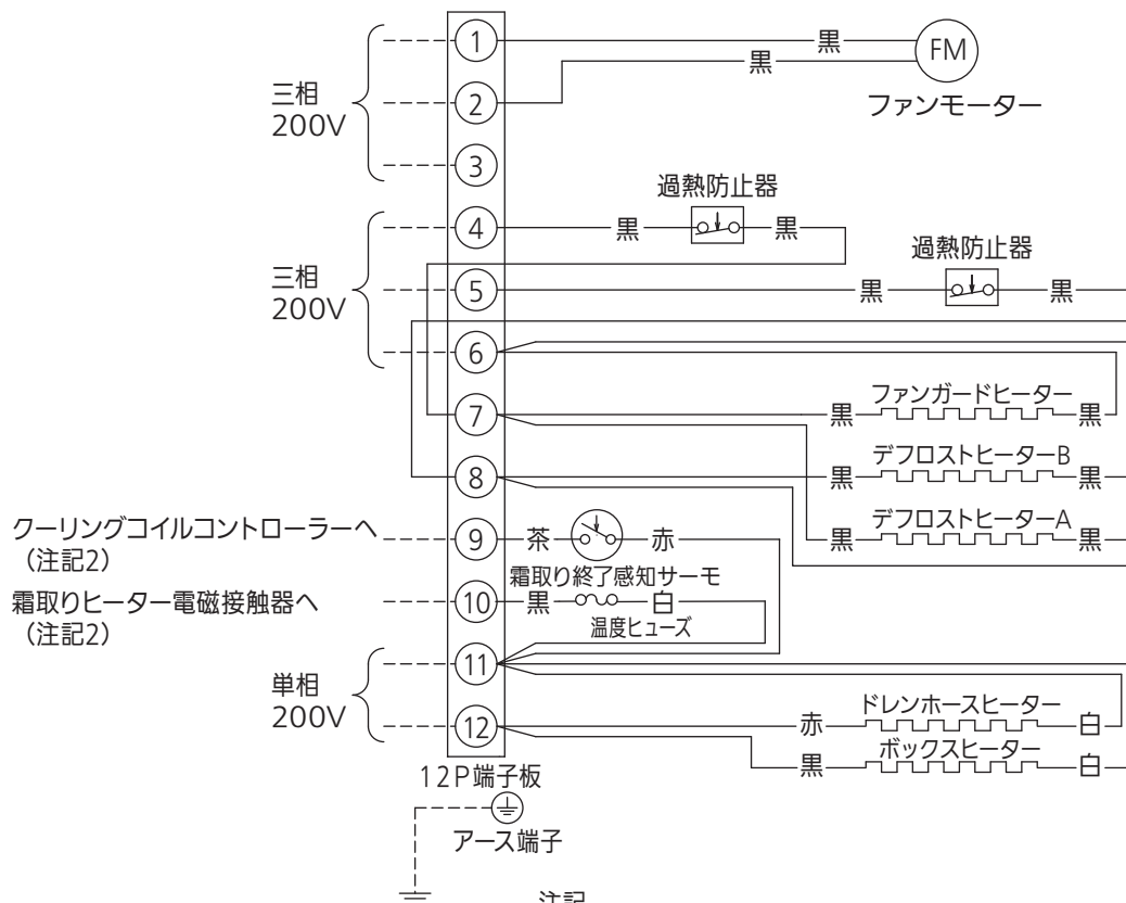
冷凍用電気回路図
