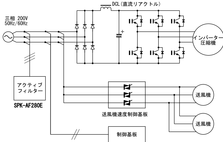
機器の基本回路図
