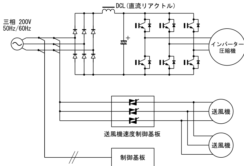
機器の基本回路図
