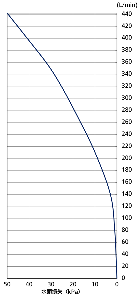
冷却水流量
