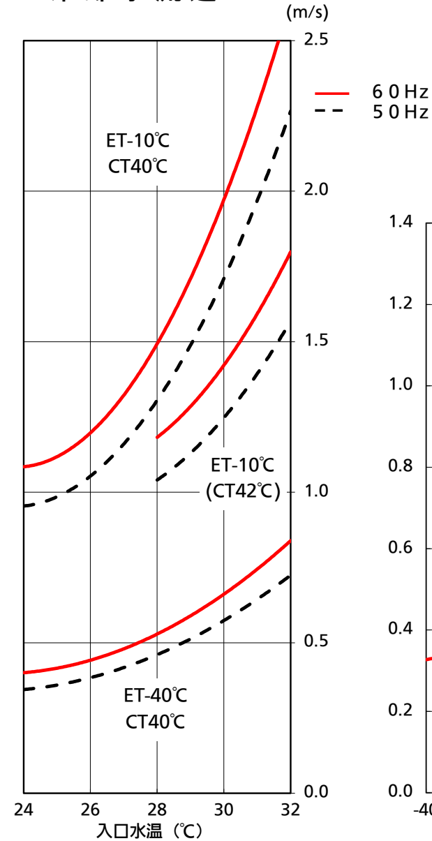
冷却水流速
