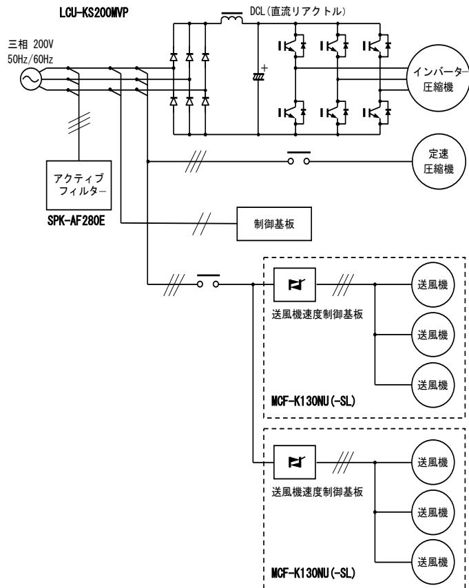
機器の基本回路図
