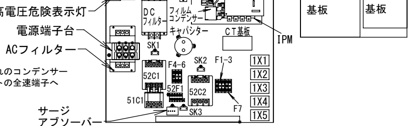
電装箱内部部品配置図 (基板を外した状態)
