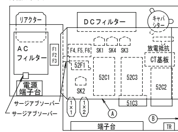
部品配置図
