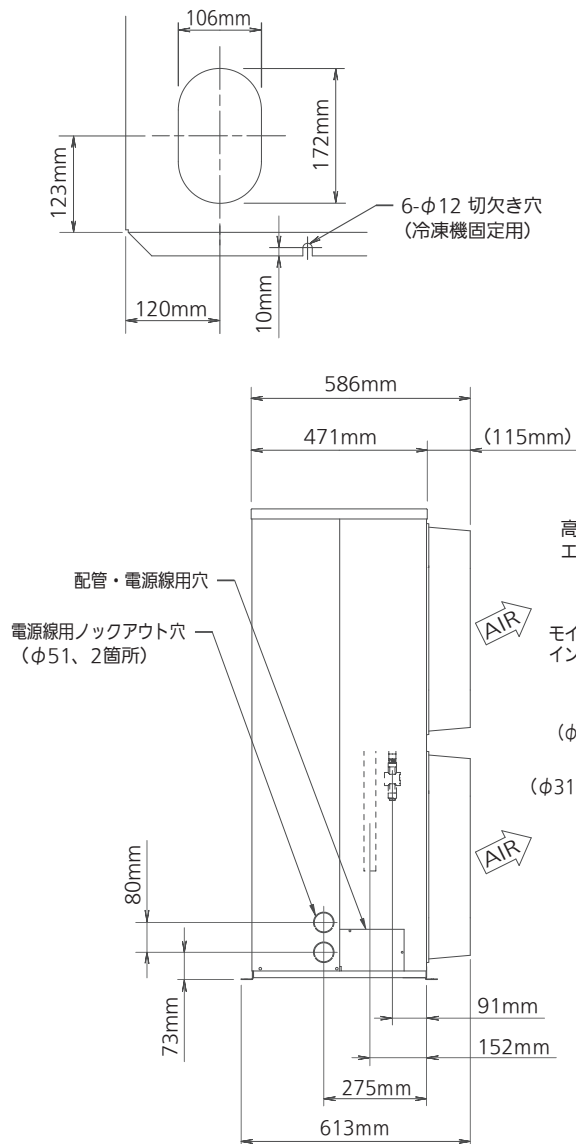
冷凍機下面配管用穴 詳細 (A部拡大図)
