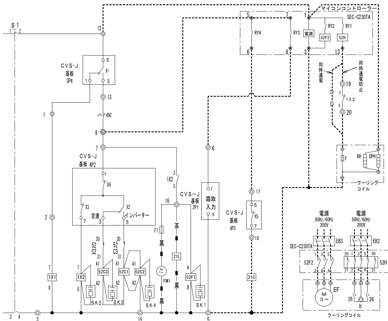
クーリングコイルとの接続例
