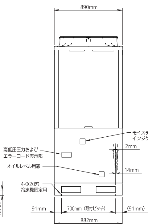
冷凍機正面
