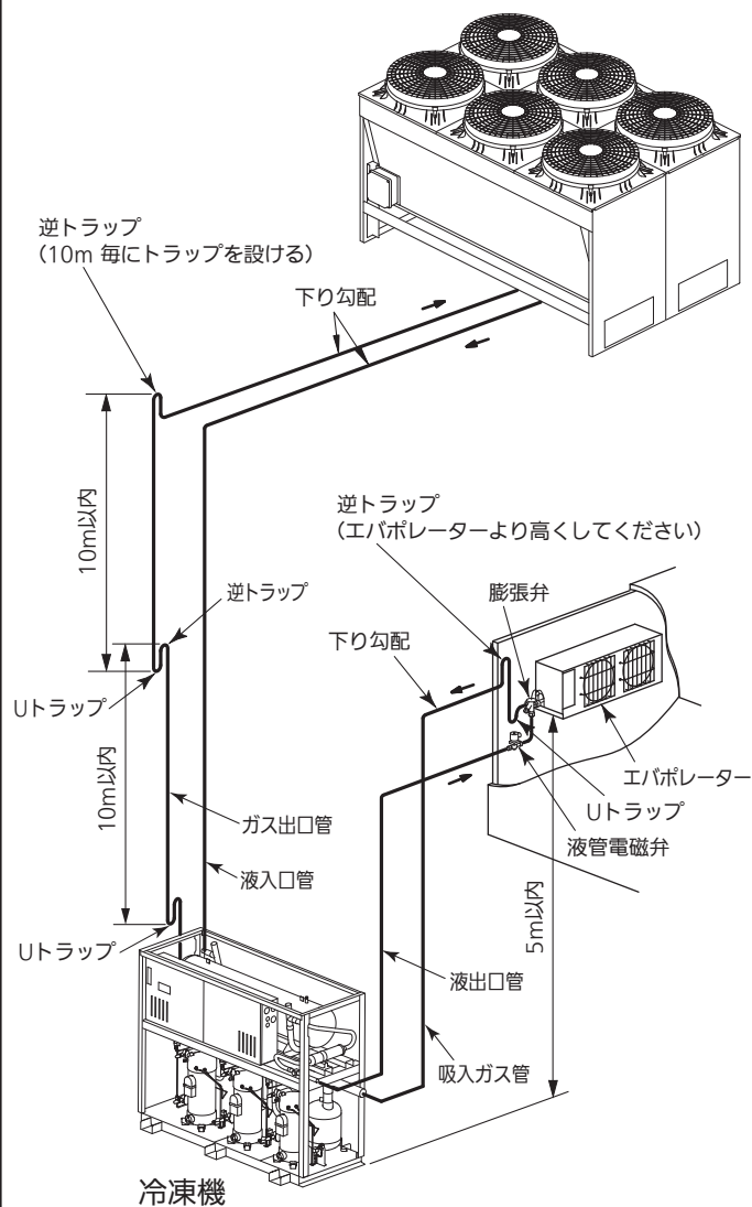
コンデンサーユニット
