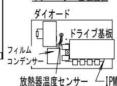
インバーター基板裏側
