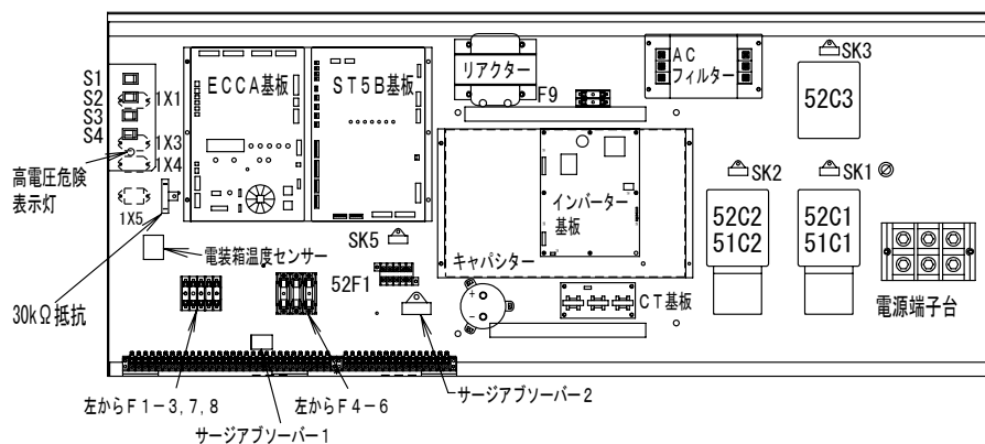
電装箱内部品配置図
