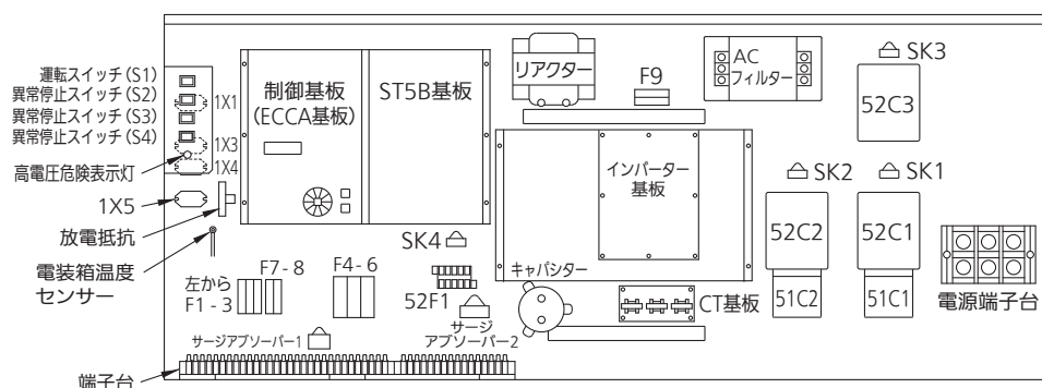
インバーター部の電気部品配置図
