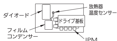
インバーター基板の裏側
