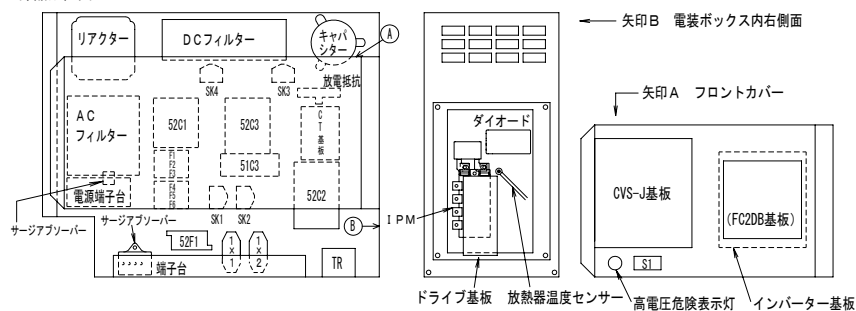
部品配置図
