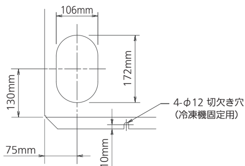
冷凍機下面配管用穴 詳細 (A部拡大図)
