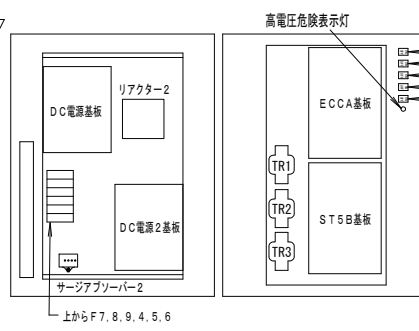
冷凍機正面裏
