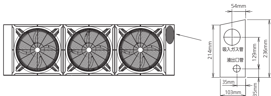
冷凍機下面配管用穴 詳細
