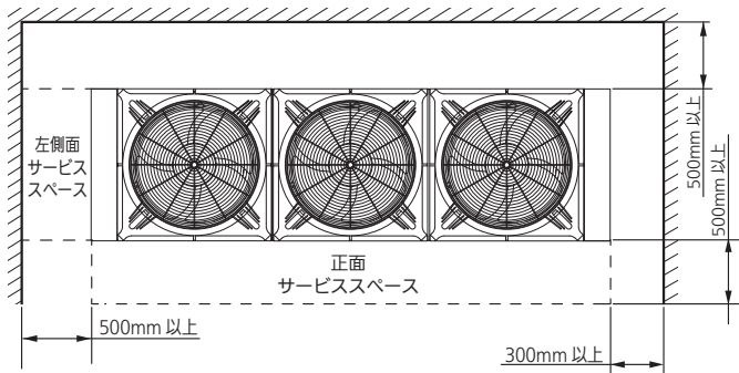
●壁が三面の場合
