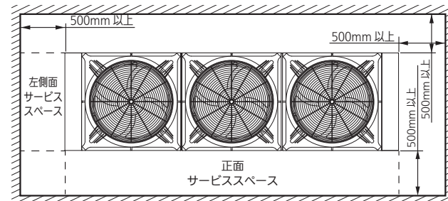
●壁が四面の場合
