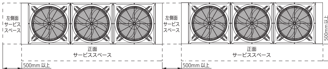
●連続設置の場合
