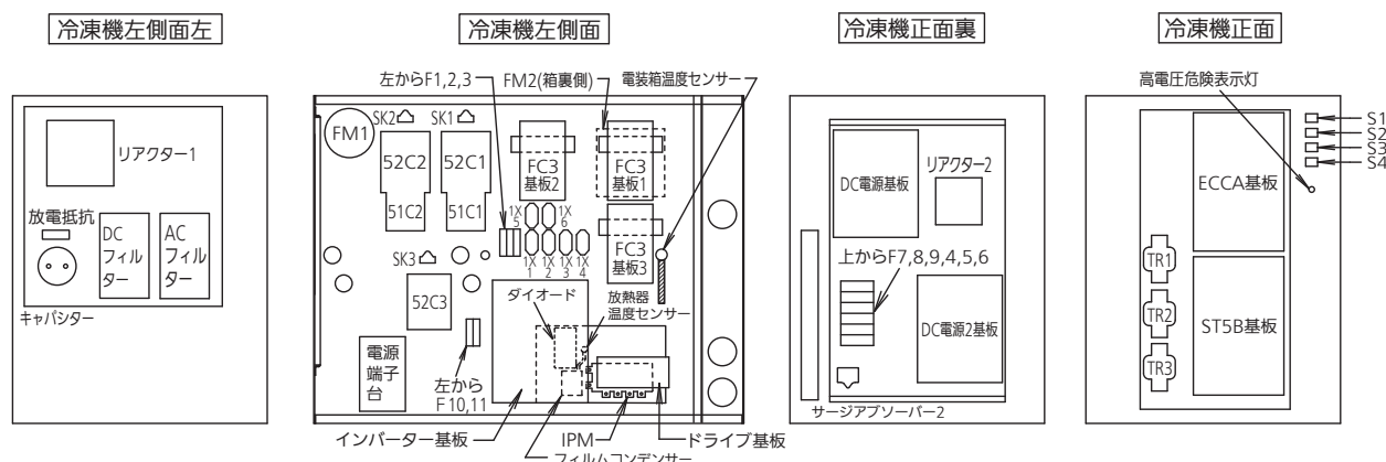
インバーター部の電気部品配置図
