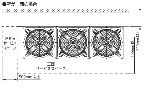
●壁が一面の場合
