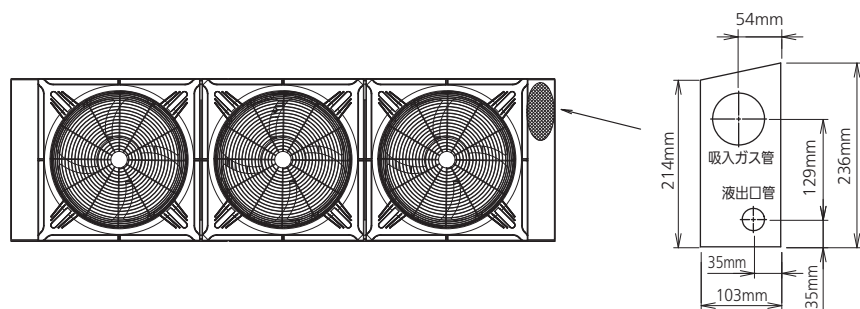
冷凍機下面配管用穴 詳細
