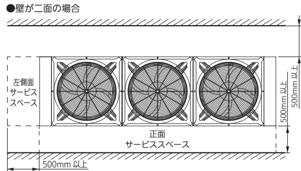
●壁が二面の場合
