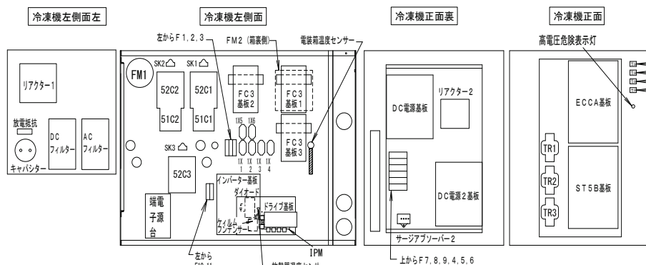
電装箱内部部品配置図
