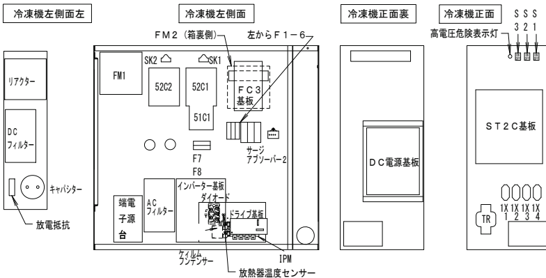
電装箱内部部品配置図
