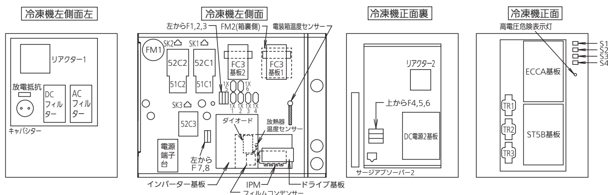
インバーター部の電気部品配置図
