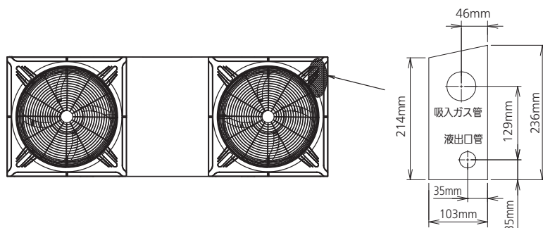
冷凍機下面配管用穴 詳細
