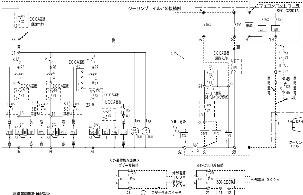
電装箱内部部品配置図
