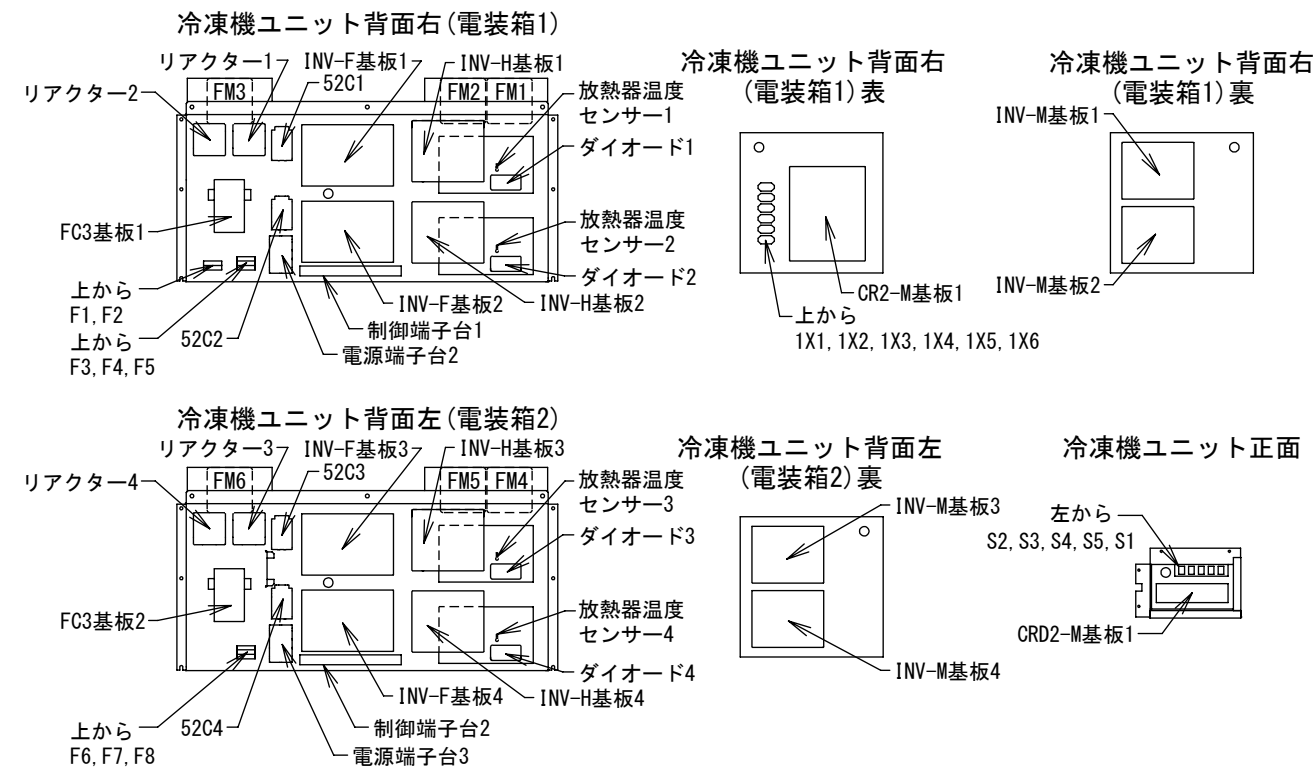
電装箱内部部品配置図 (冷凍機ユニット側)
