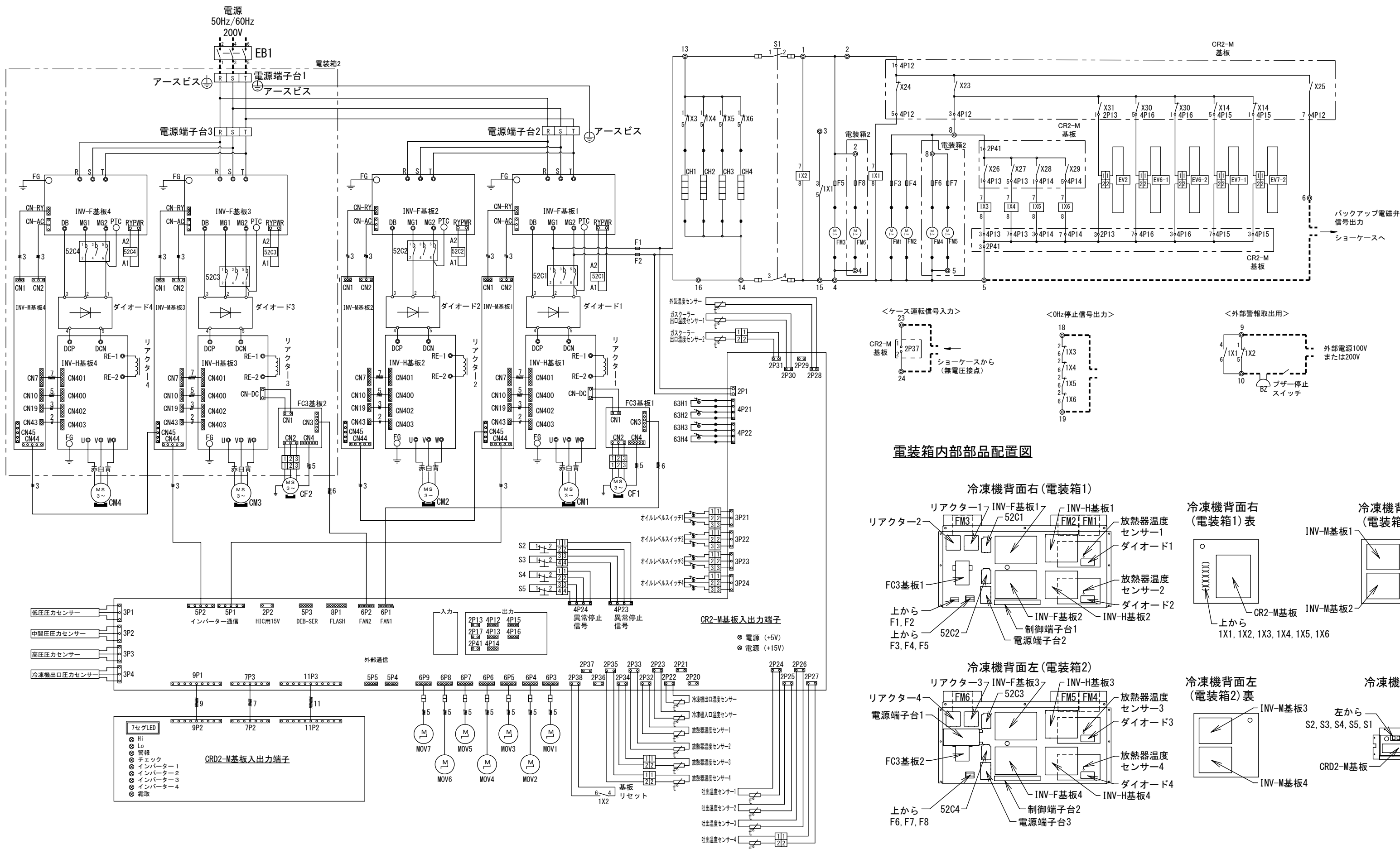
推奨回路図 (OCU-CR4000MVF)
