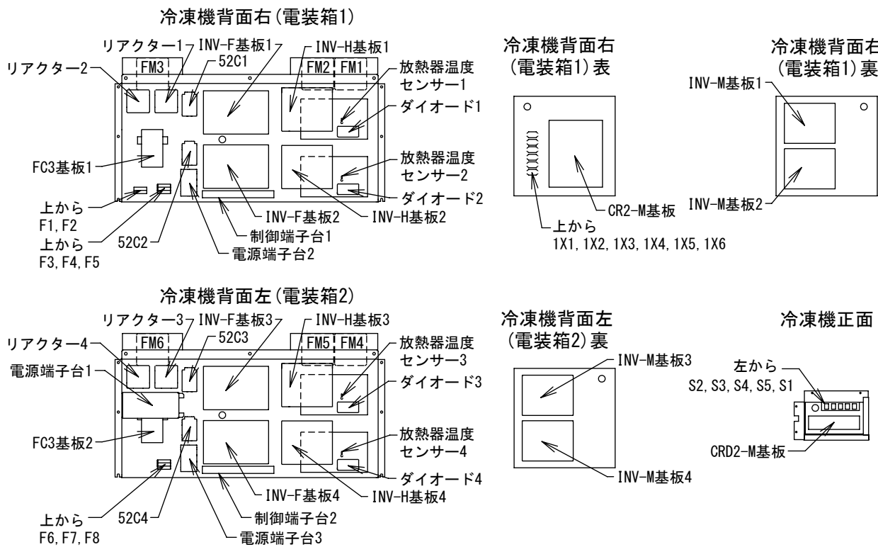
電装箱内部部品配置図
