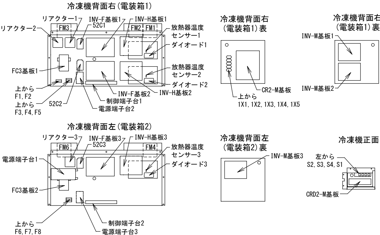
配置図電装箱内部部品配置図
