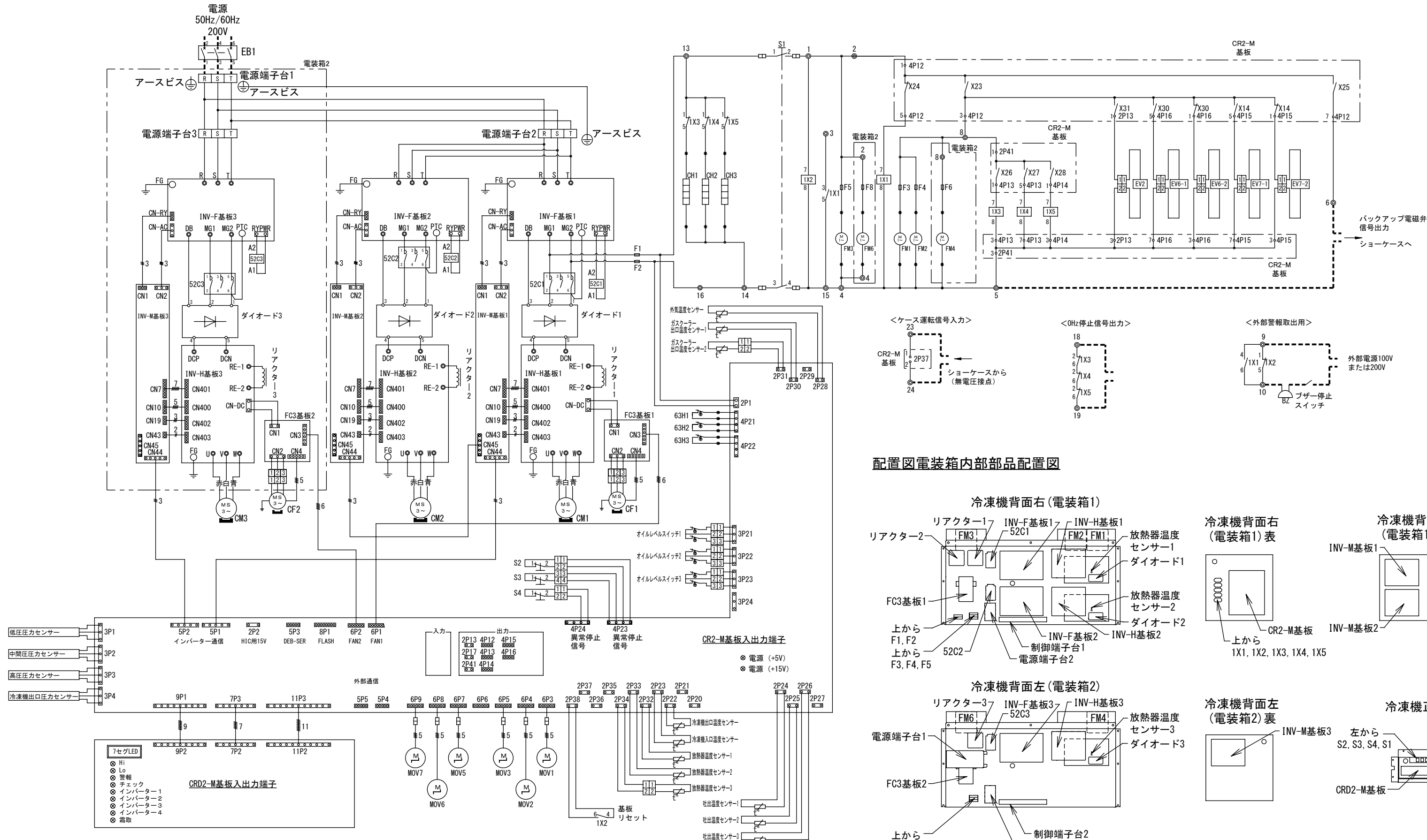
推奨回路図 (OCU-CR3000MVF)
