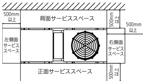
＜ 壁が一面の場合 ＞
