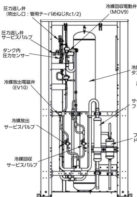
タンクユニット左側面
