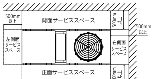
＜ 壁が四面の場合 ＞
