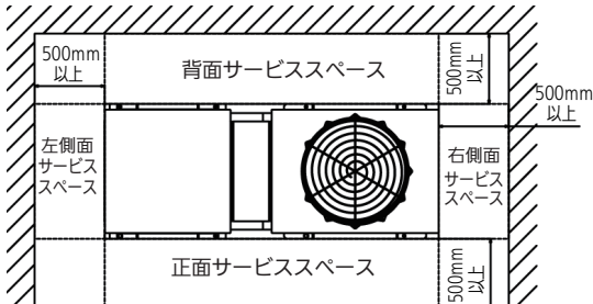
＜ 壁が四面の場合 ＞
