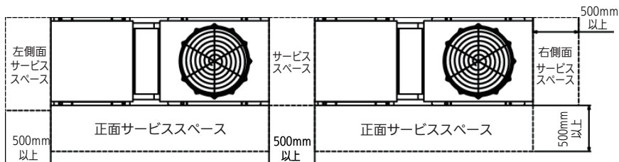
＜ 連続設置の場合 ＞
