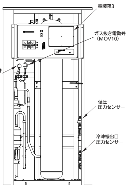
タンクユニット正面
