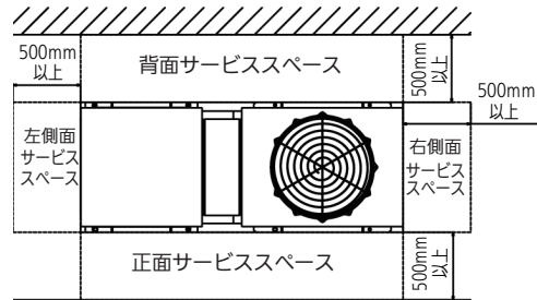
＜ 壁が二面の場合 ＞
