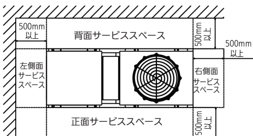
＜ 壁が三面の場合 ＞
