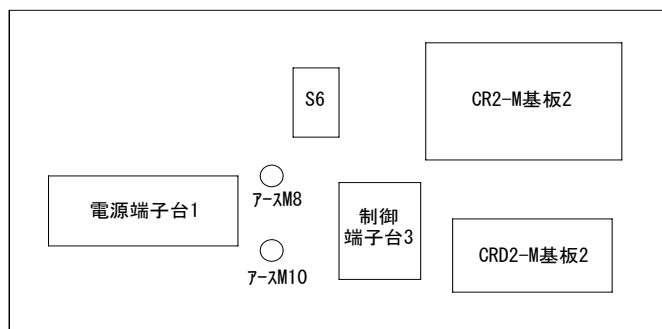
電装箱 3 の内部部品配置図（タンクユニット側）
