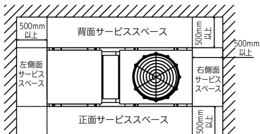
＜ 壁が三面の場合 ＞
