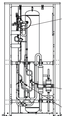
タンクユニット左側面
