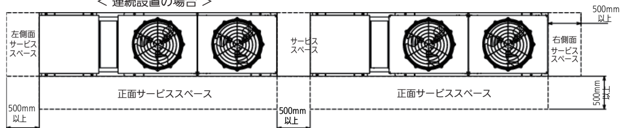
< 連続設置の場合 >
