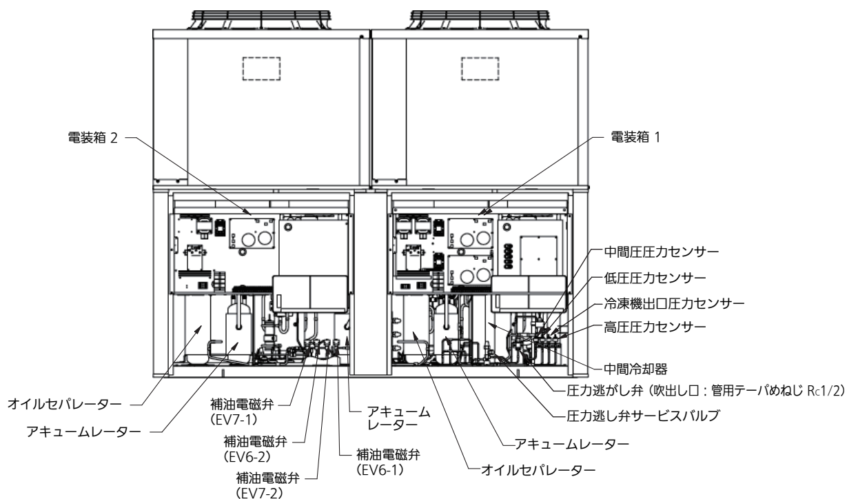
冷凍機ユニット背面
