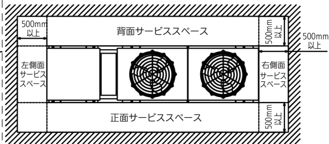
< 壁が四面の場合 >
