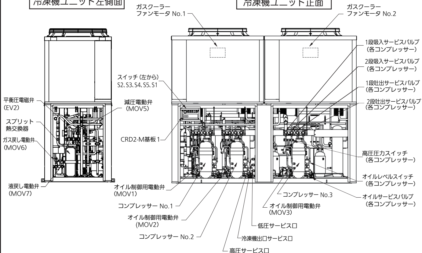
冷凍機ユニット左側面
