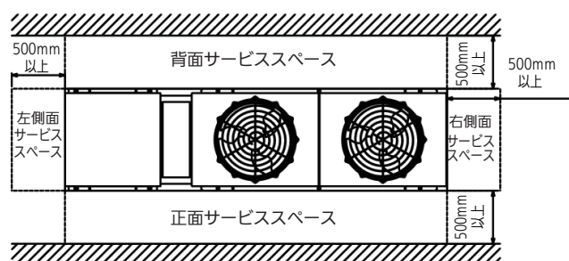
< 壁が二面の場合 >
