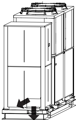
冷凍機左側面
