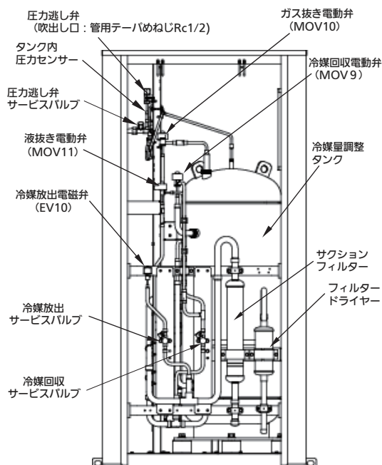
タンクユニット左側面
