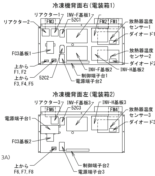
配置図電装箱内部部品配置図
