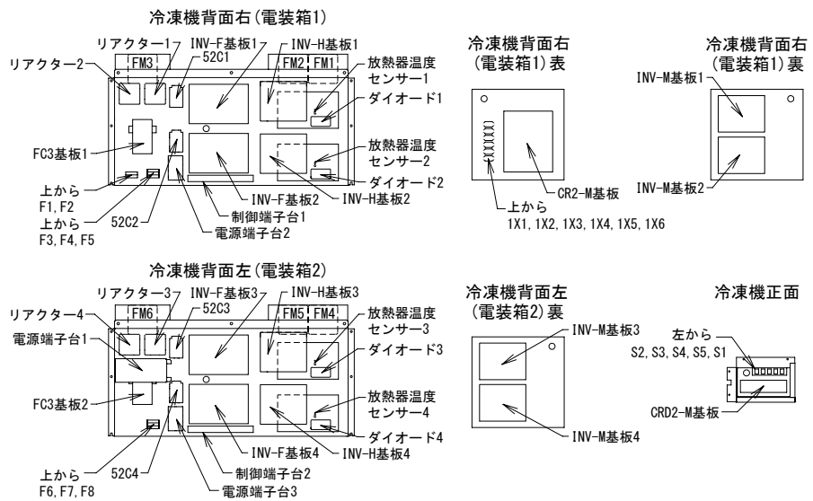
電装箱内部部品配置図
