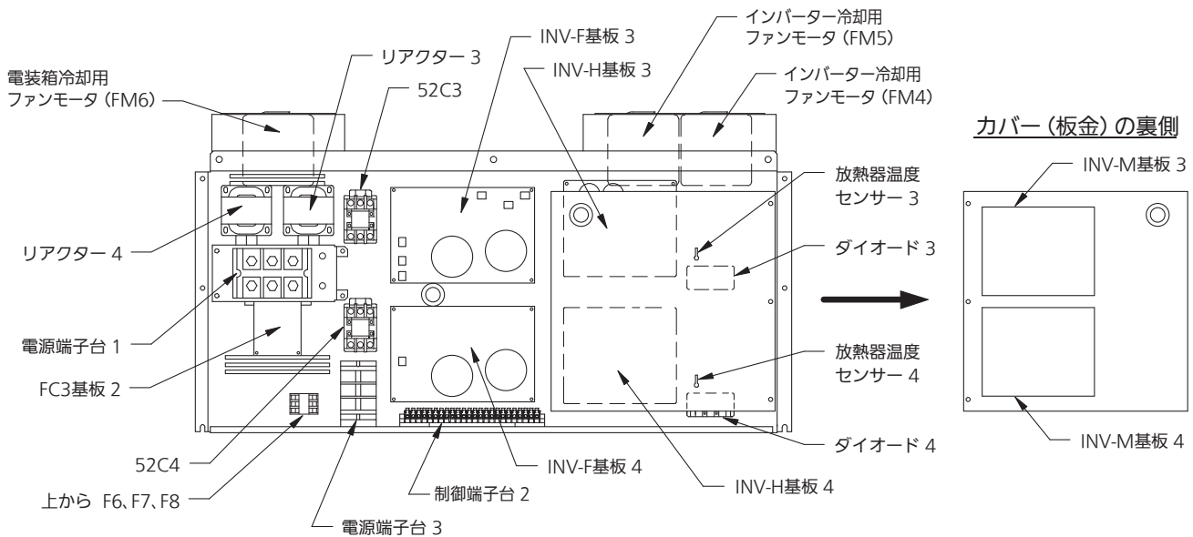
冷凍機背面左 <電装箱 2>
