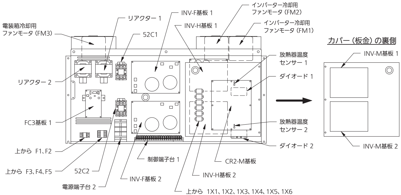
冷凍機背面左 <電装箱 2>
