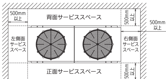
＜ 壁が三面の場合 ＞
