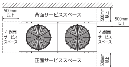
＜ 壁が一面の場合 ＞
