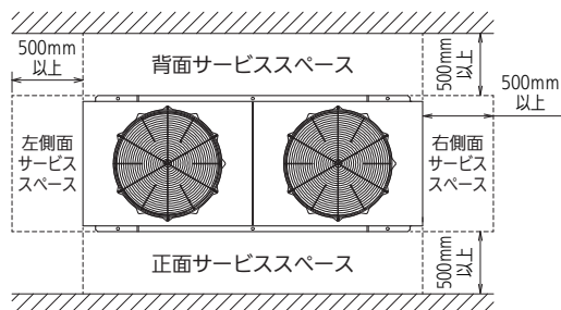
＜ 壁が二面の場合 ＞
