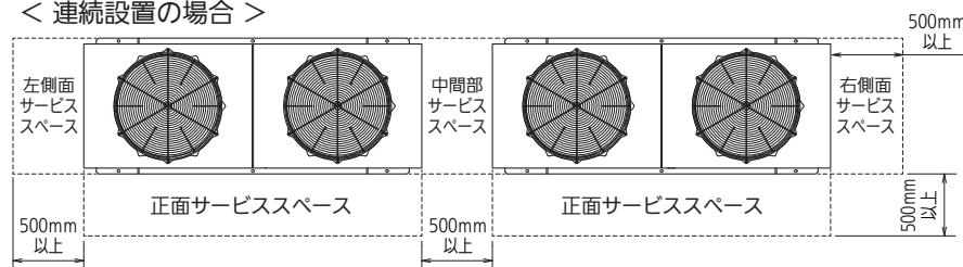
＜ 連続設置の場合 ＞
