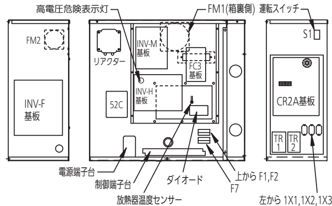
冷凍機左側面左
