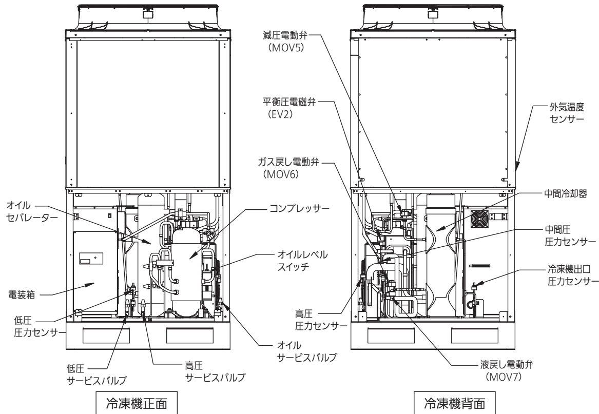
電装箱内部配置図
