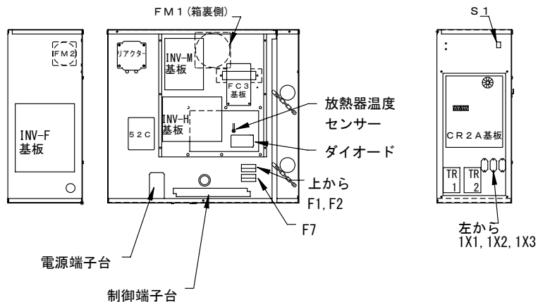
電装箱内部部品配置図
