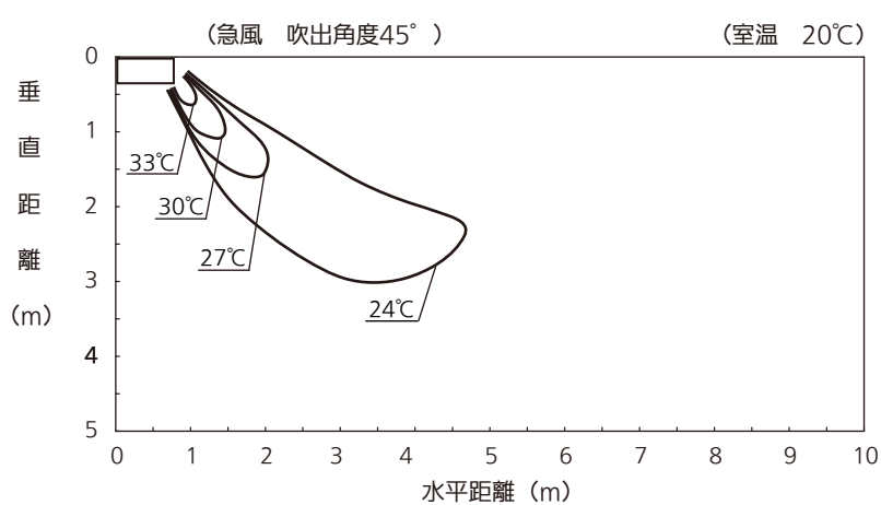
暖房 温度分布
