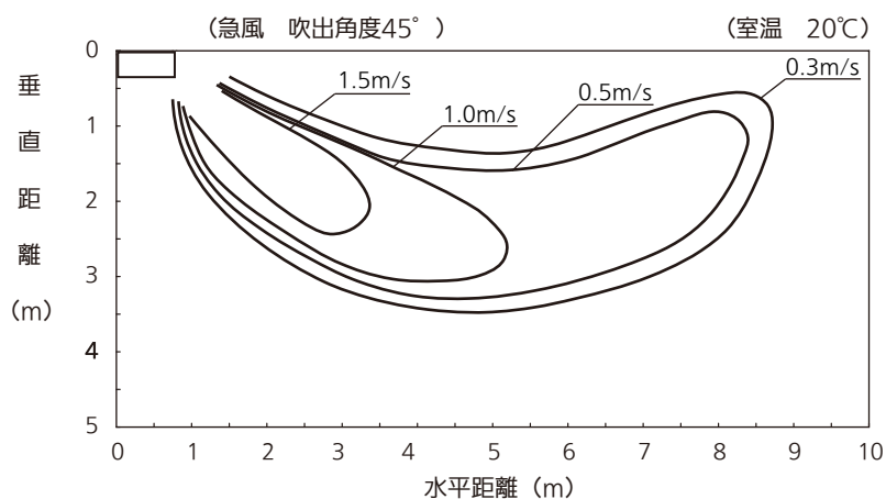
暖房 風速分布
