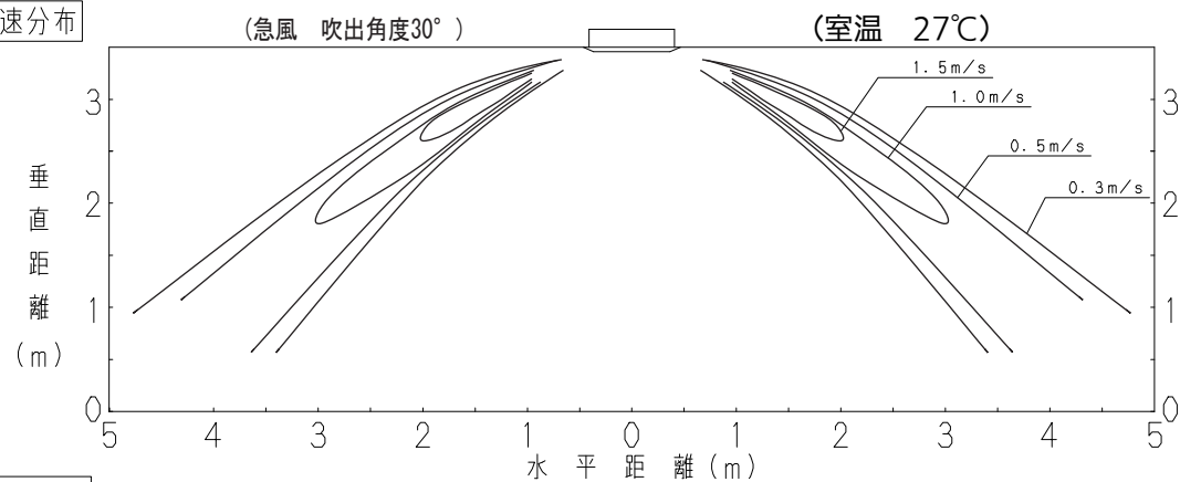
冷房 温度分布
