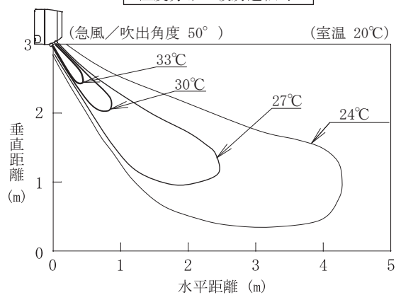
温度分布《冷房運転時》
