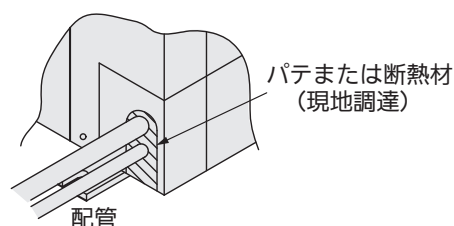
小動物侵入防止対策 図 2
