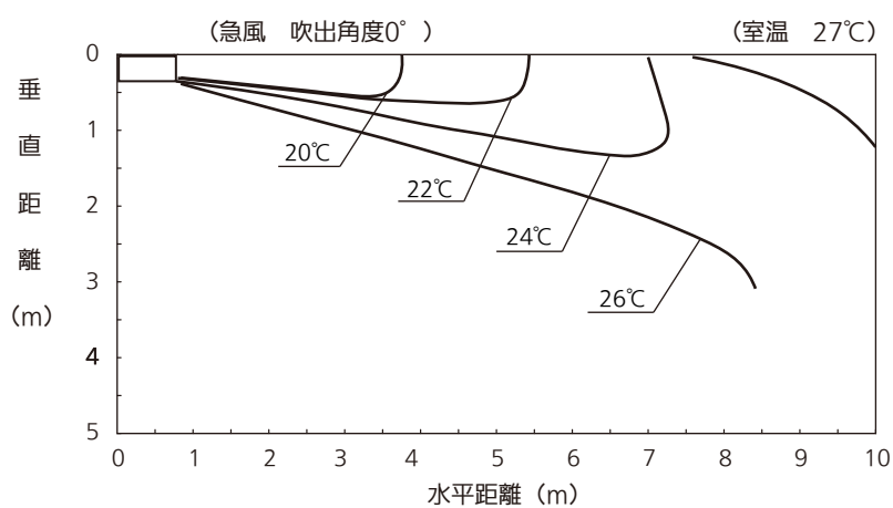
冷房 温度分布
