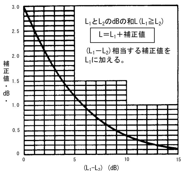
(図6) 合成音の補正值
