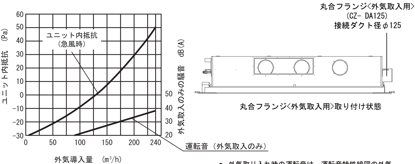
外気導入量とユニット内抵抗・運転音特性
