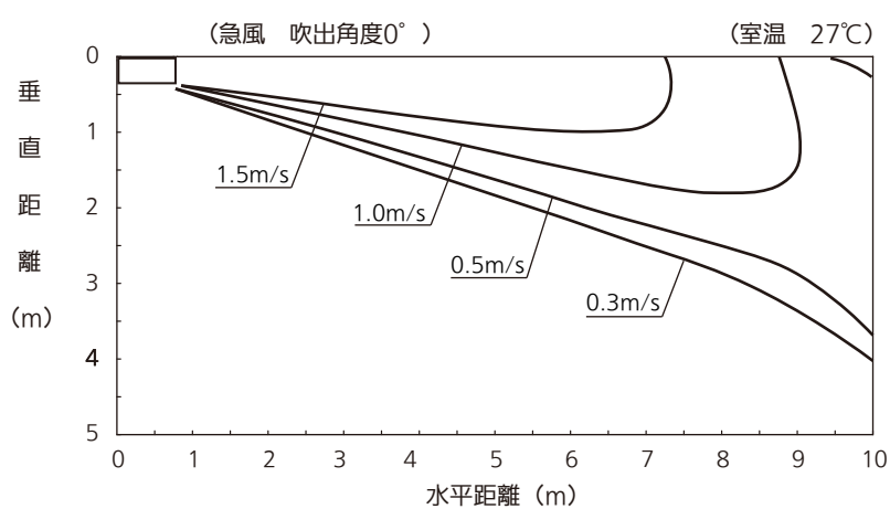
冷房 風速分布
