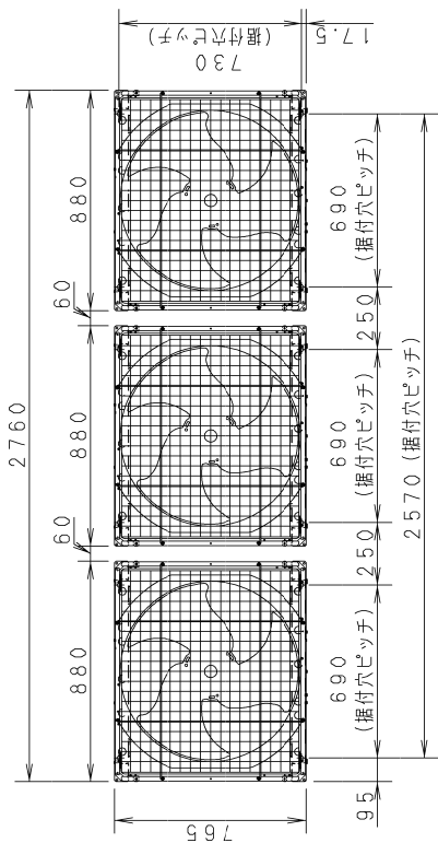
天面
