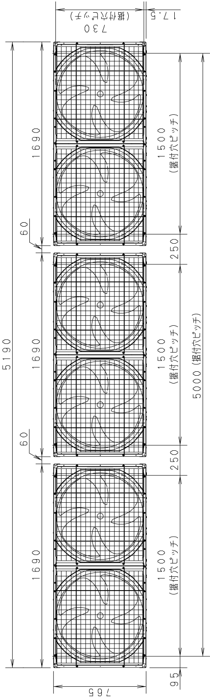
天面
