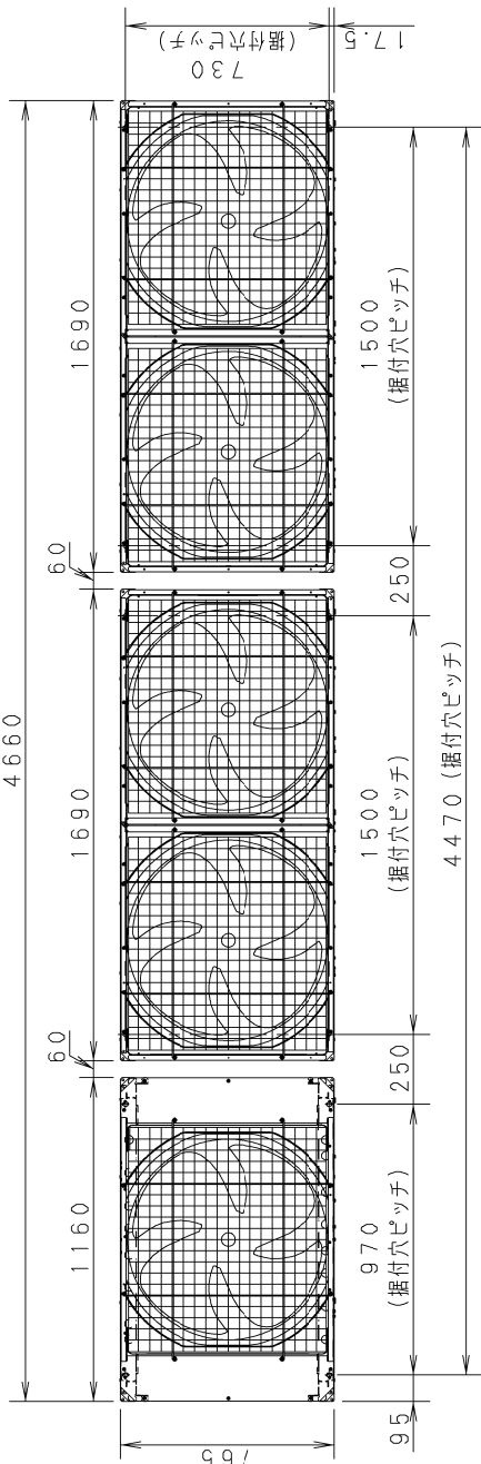
天面
