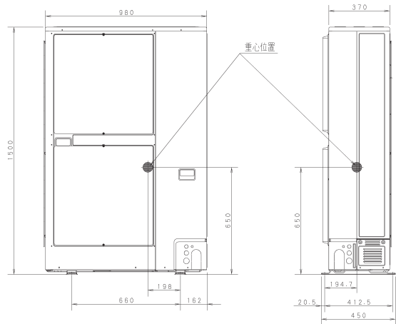
外観略図 CU-P112,P140,P160UL4R
