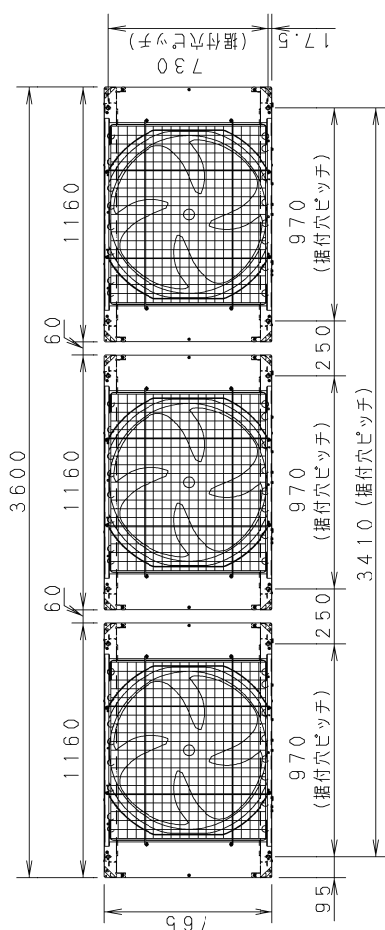
天面
