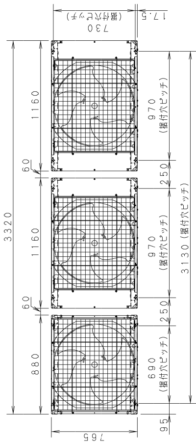
天面
