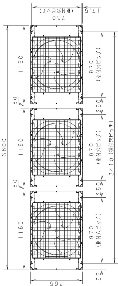
天面
