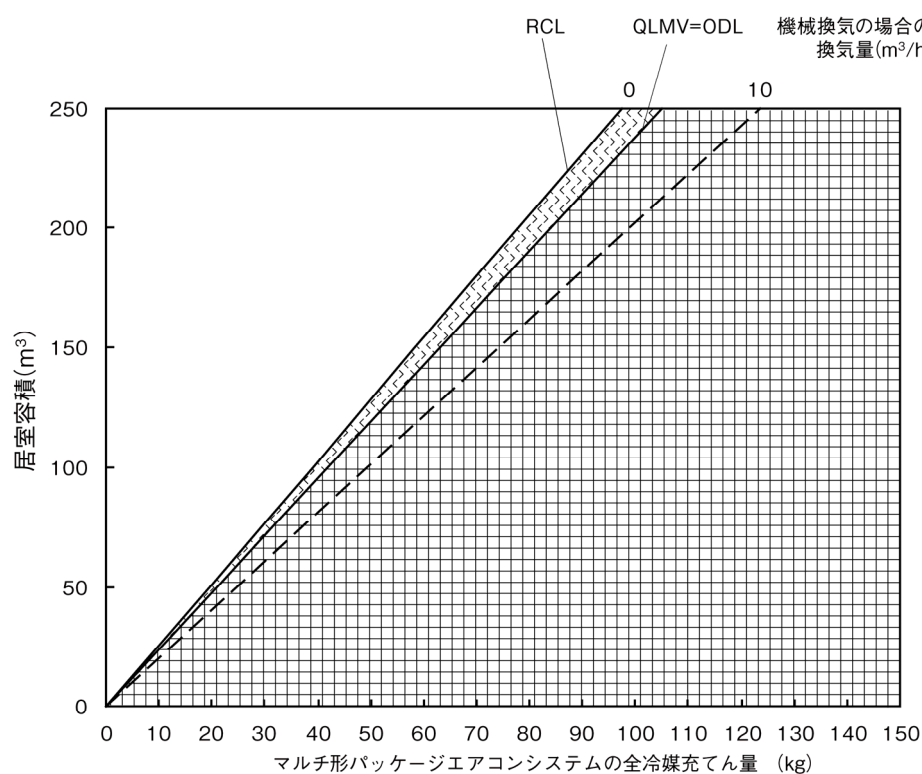
図 6 ー 特定システムの許容冷媒充てん量と必要な対策 [R410A 冷媒] <地下の最下層階の場合>
