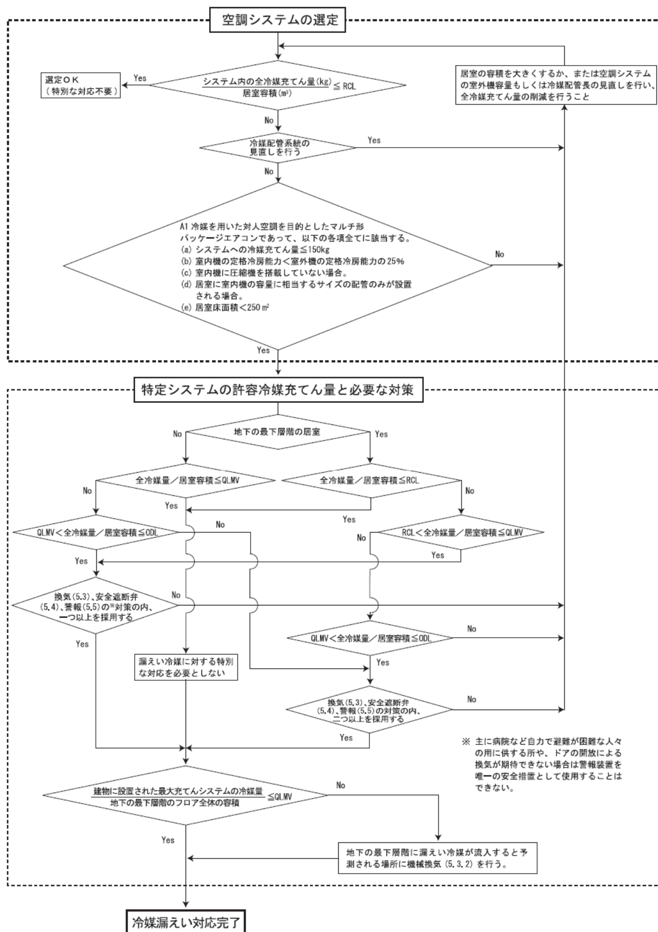
図 2 - 冷媒漏えい対応フローチャート
