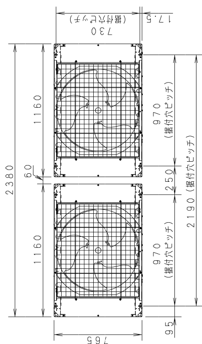
天面
