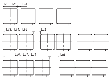
＜第5図＞U×KR5シリーズ 室外ユニットの設置寸法（ブロック間の距離）
