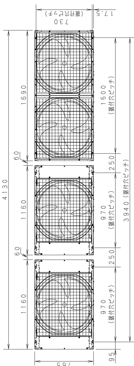
天面
