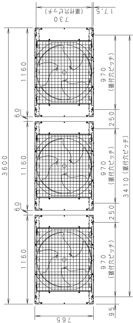
天面
