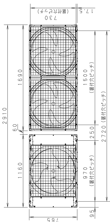
天面
