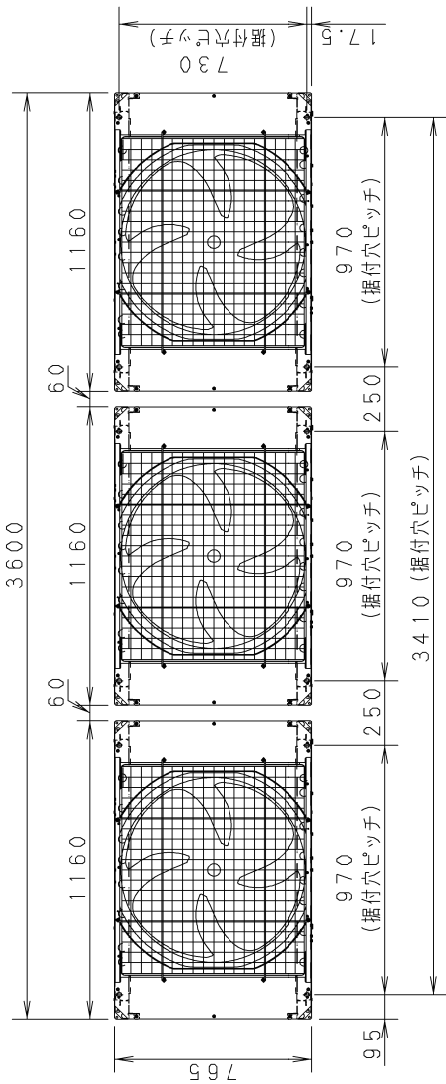
天面
