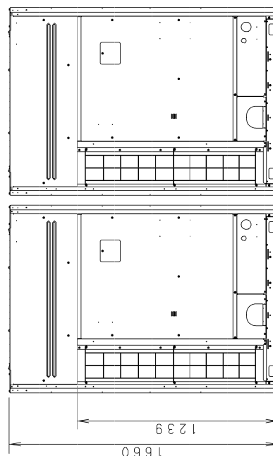
正面
