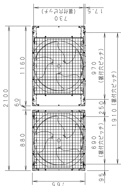
天面
