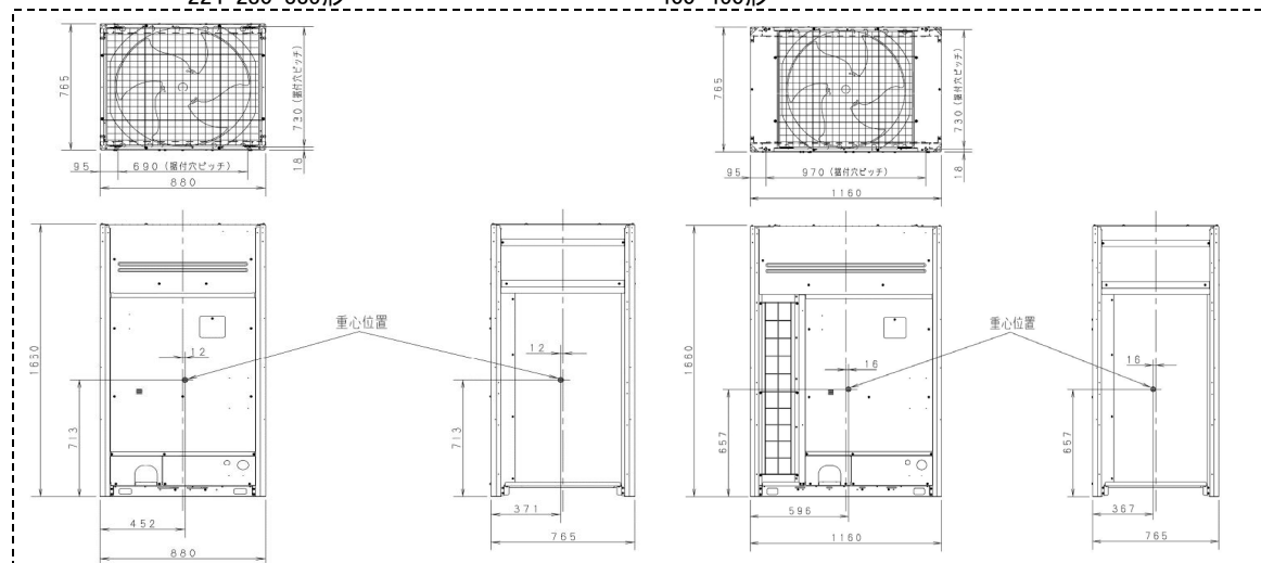
外観略図
