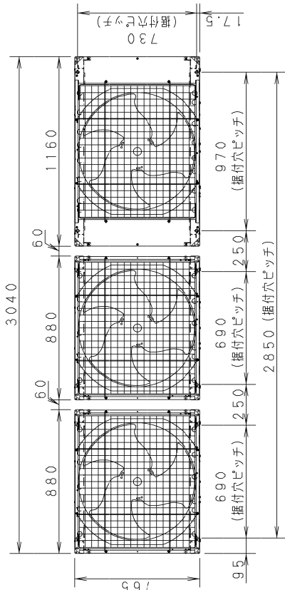
天面
