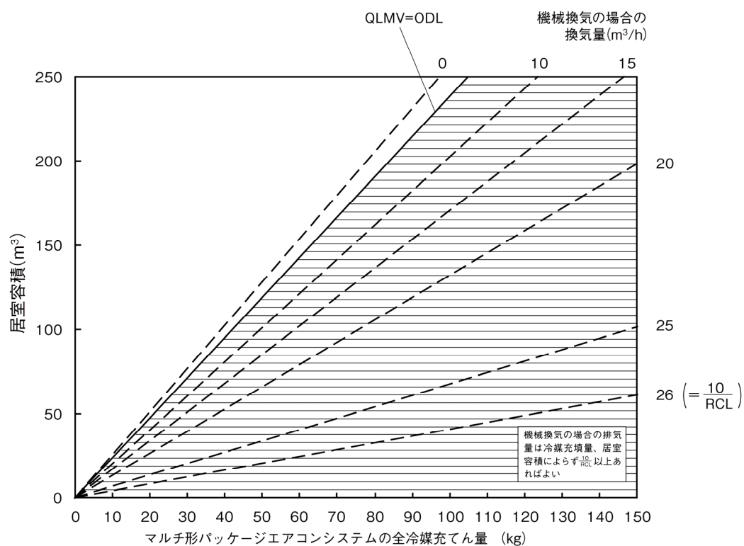
図 5 ー 特定システムの許容冷媒充てん量と必要な対策 [R410A 冷媒] <地下の最下層階以外の場合>
