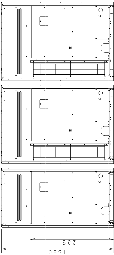
正面
