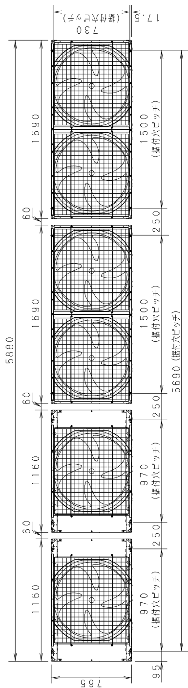
天面
