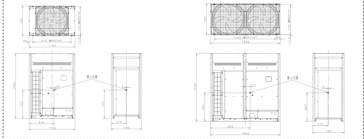
外観略図 160・224形
