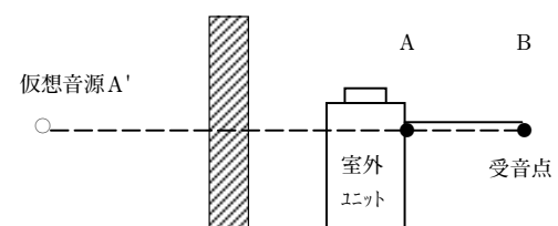
(図5)反射音増加(壁面)
