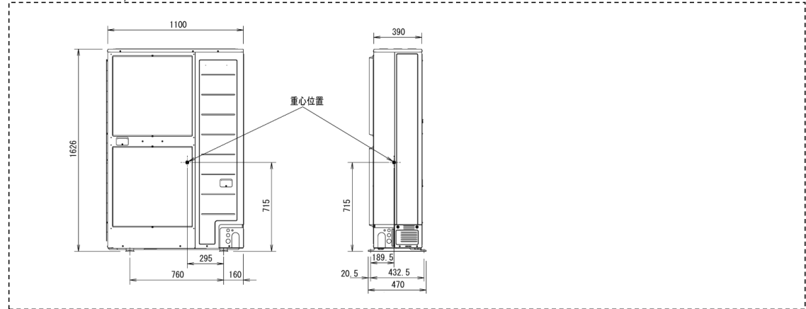
外観略図 CU-P224,280ULR5R
