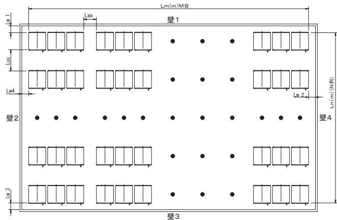
＜第1図＞室外ユニット集合時設置時の寸法
