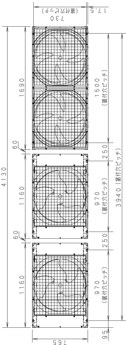
天面
