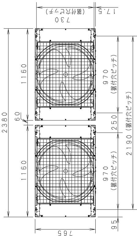
天面
