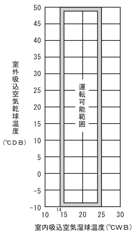
冷房時の使用限界
