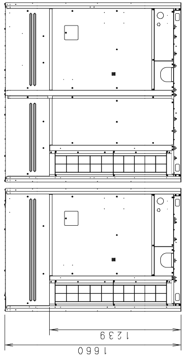
正面
