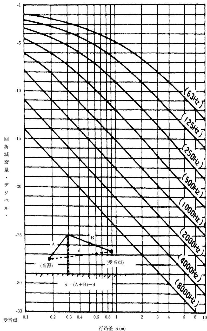
(図2)回折減衰量
