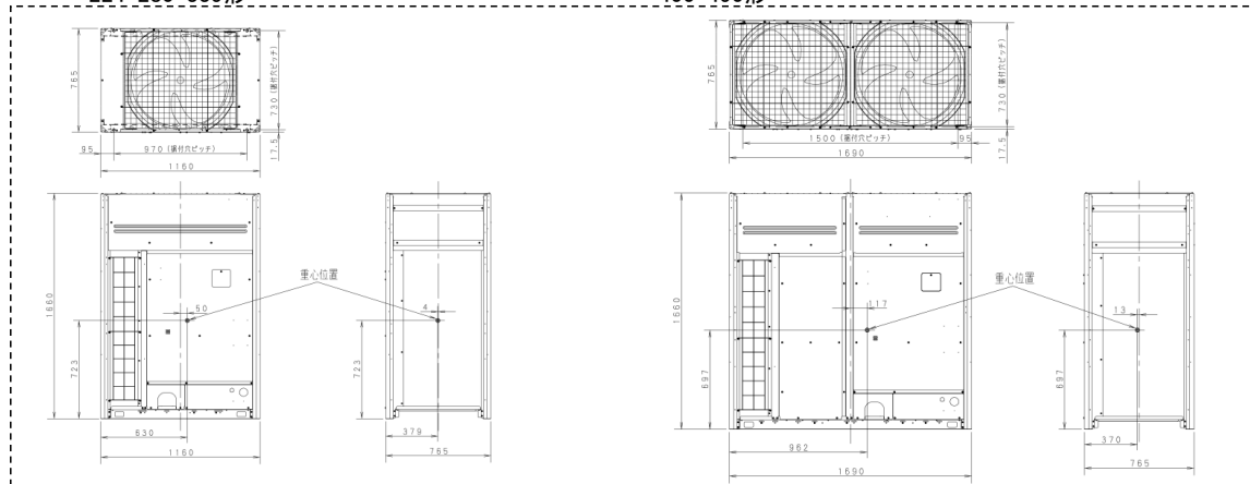
外観略図
