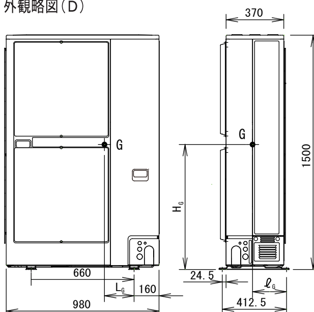
外観略図(D)
