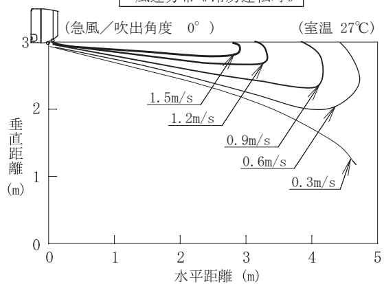
風速分布《冷房運転時》
