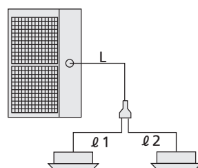
室内ユニット(56形×2台)
