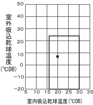
10°Cタイプ暖房時
