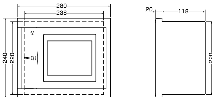
外形寸法図
