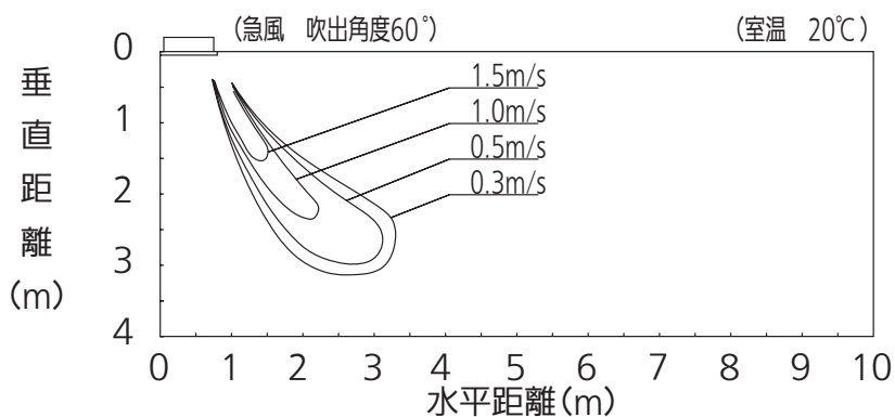
暖房 風速分布
