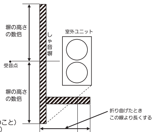
図4 しゃ音塀
