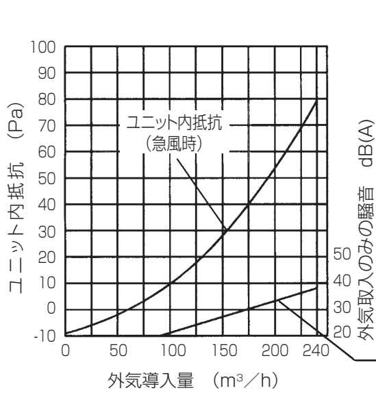
外気導入量とユニット内抵抗・運転音特性 ※ 急風：風速5速中最大（レベル5）
