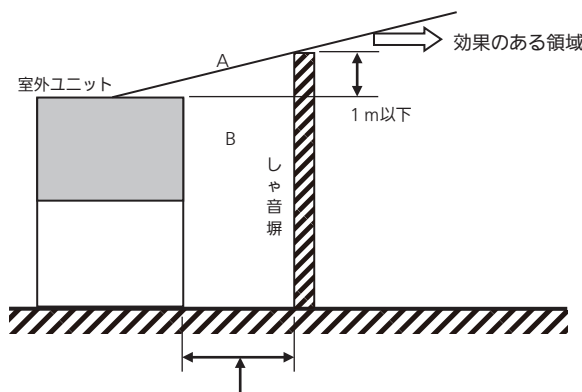
図3 しゃ音塀
