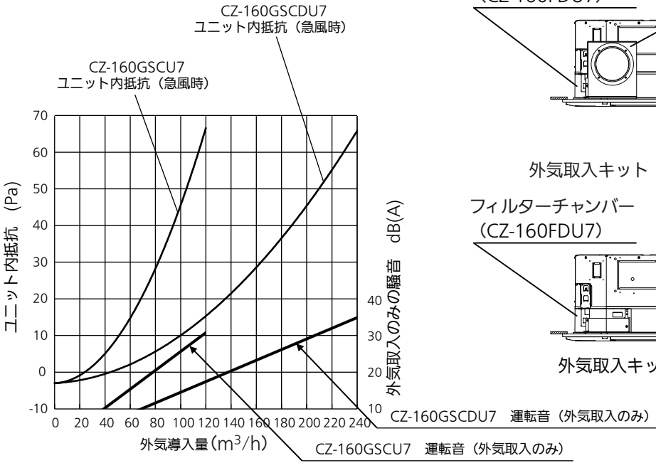
外気導入量とユニット内抵抗・運転音特性 ※ 急風：風速5速中最大 (レベル5)
