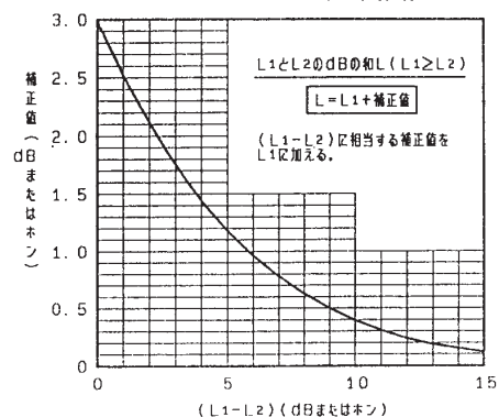
図5 合成音の補正值
