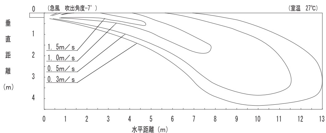
冷房 風速分布
