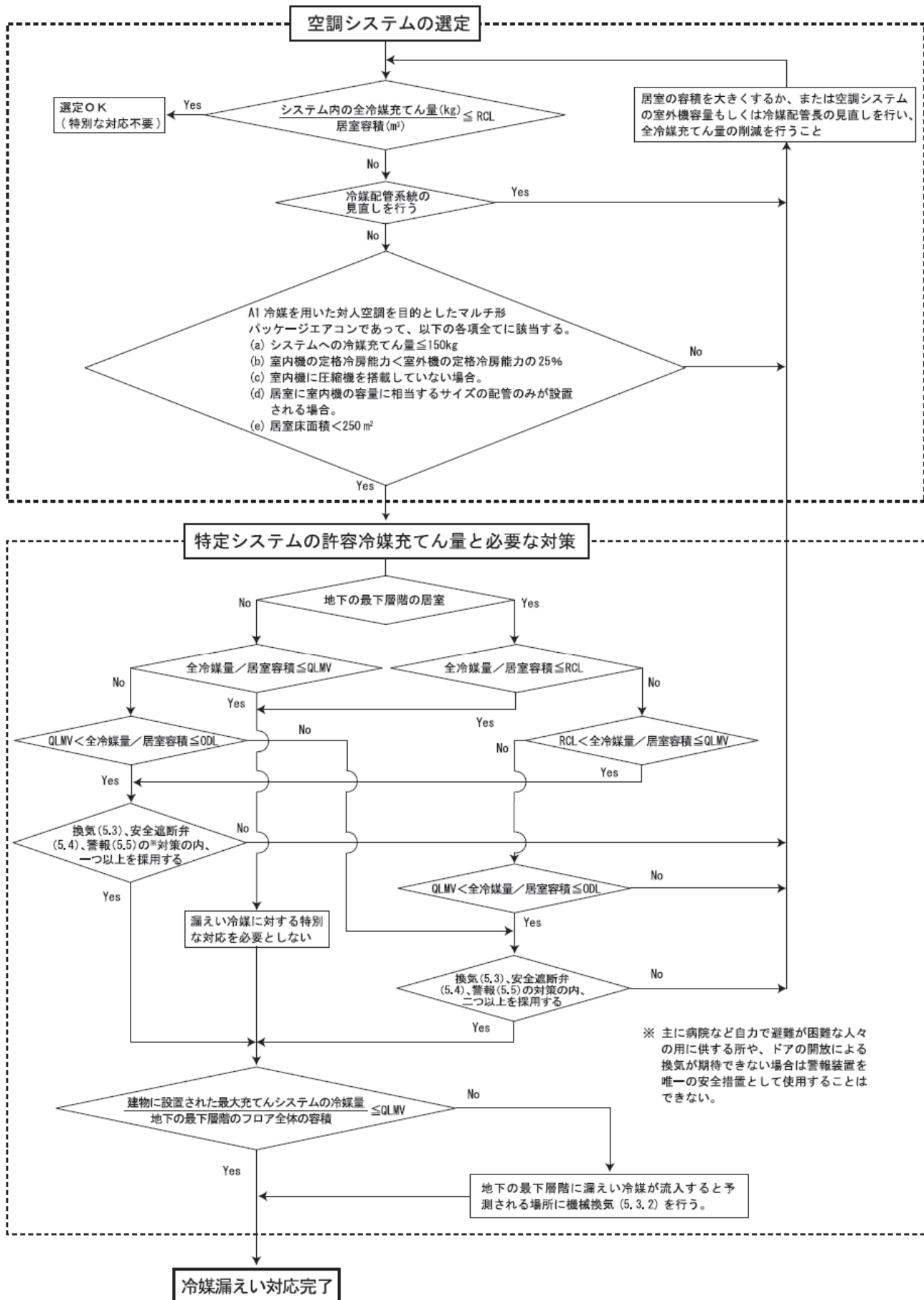
図3 冷媒漏えい対応フローチャート
