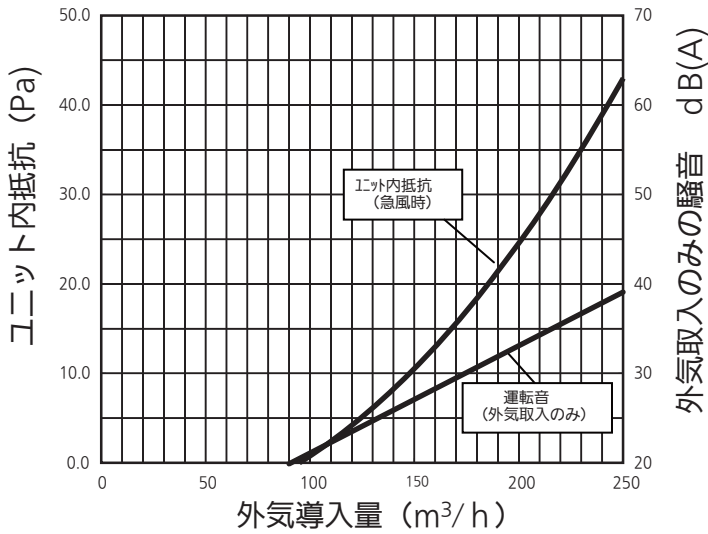
外気導入量とユニット内抵抗・運転音特性
